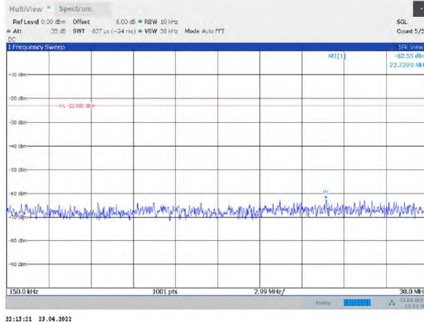
Band43-20MHz-QPSK-44690-1RB#0-Range2:0.15~30MHz
