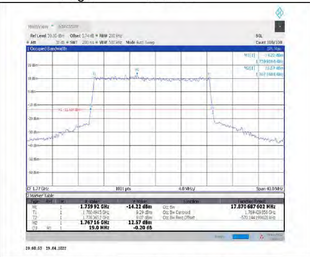
1-N66-PC3-15-20-H-3-DFT-16QAM-Outer_Full-100@0-Ant1-17.871-19.000-≤20-PASS
