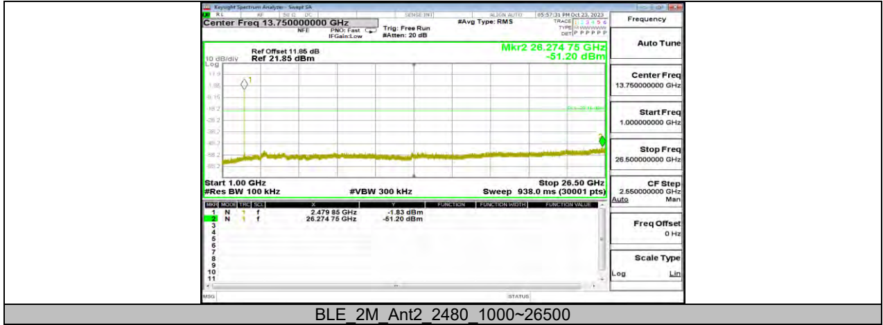
BLE_2M_Ant2_2480_1000~26500
