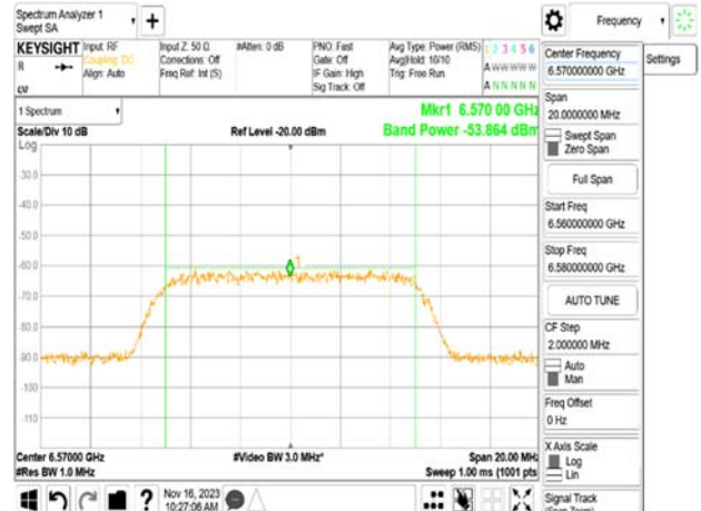
FMCW_150MHz_6500MHz_AWGN:6570MHz
