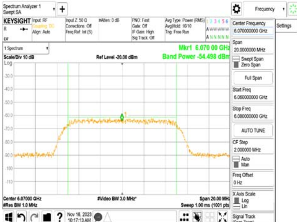
FMCW_150MHz_6000MHz_AWGN:6070MHz
