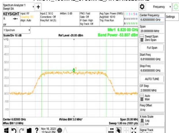
FMCW_150MHz_6750MHz_AWGN:6820MHz
