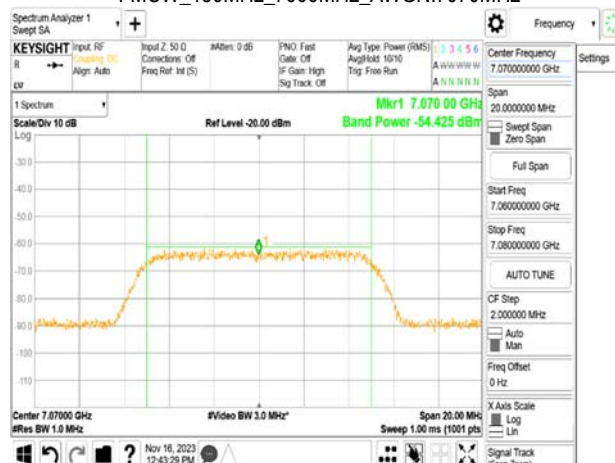
FMCW_150MHz_7000MHz_AWGN:7070MHz
