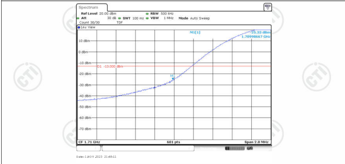
Band66-20MHz-16QAM-132072-1RB#99
