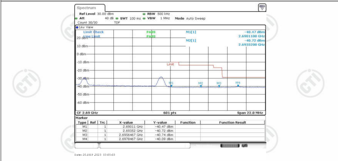
Band41-20MHz-16QAM-41490-1RB#99
