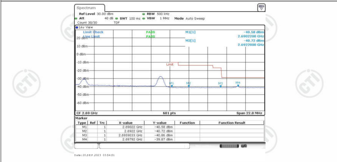
Band41-20MHz-QPSK-41490-1RB#99
