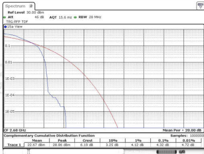
Band41-20MHz-16QAM-41490-1RB#0
