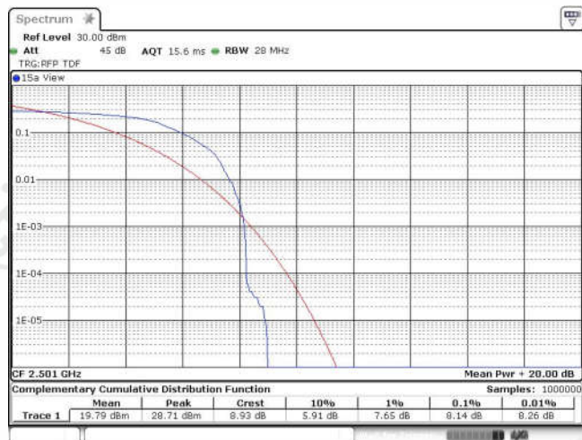
Band41-10MHz-QPSK-39700-50RB#0
