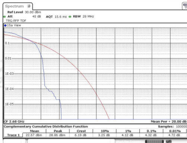
Band41-20MHz-QPSK-41490-1RB#0
