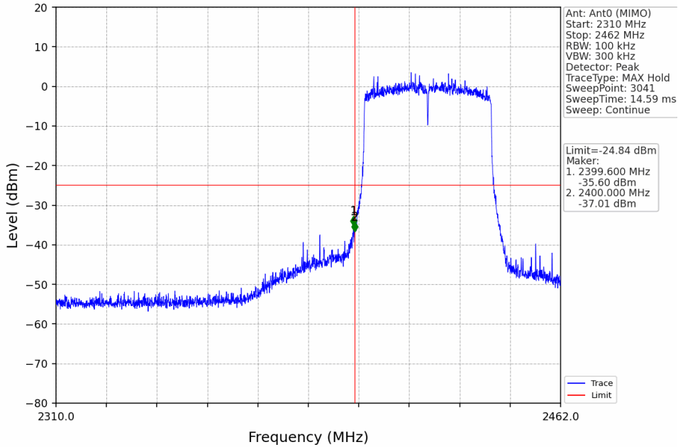
802.11ax(HEW40)_LCH_2422MHz_RU484_Left_Ant0 (MIMO)_NTNV
