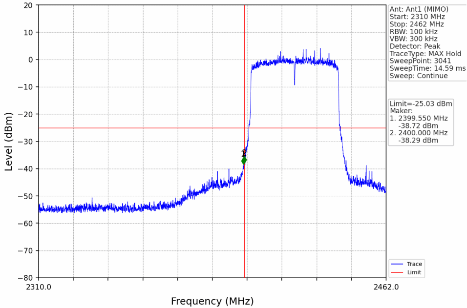
802.11ax(HEW40)_LCH_2422MHz_RU484_Left_Ant1 (MIMO)_NTNV
