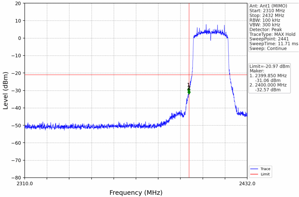
802.11ax(HEW20)_LCH_2412MHz_RU242_Left_Ant1 (MIMO)_NTNV
