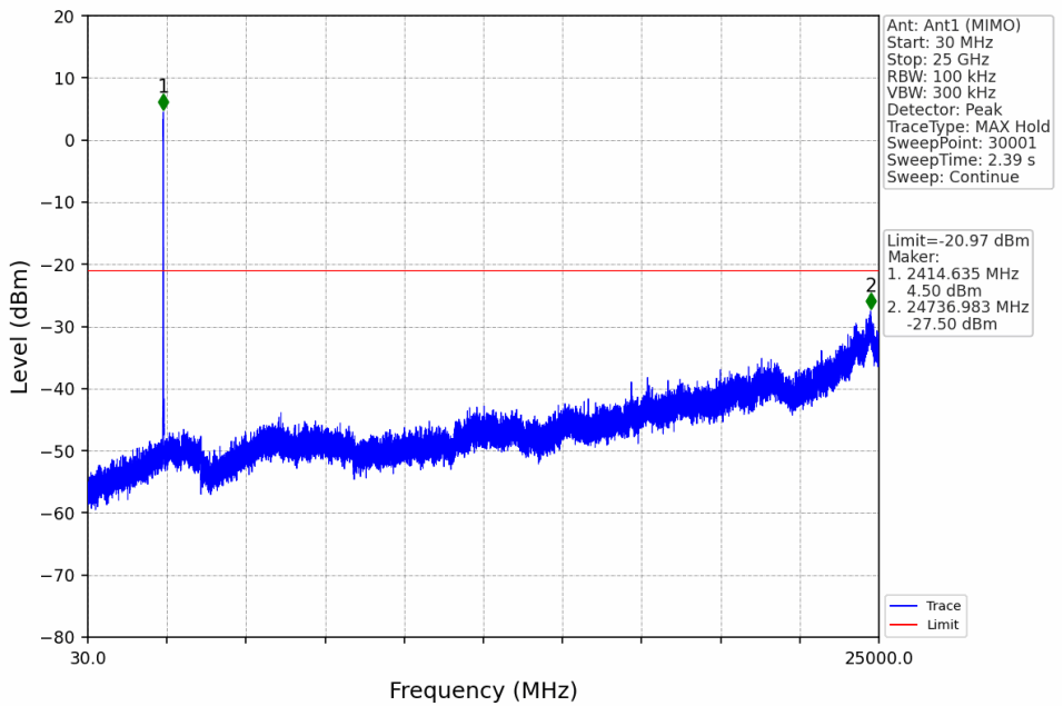
802.11ax(HEW20)_LCH_2412MHz_RU242_Left_Ant1 (MIMO)_NTNV
