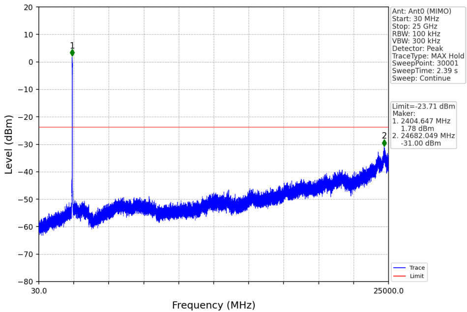
802.11n(HT40)_LCH_2422MHz_Ant0 (MIMO)_NTNV
