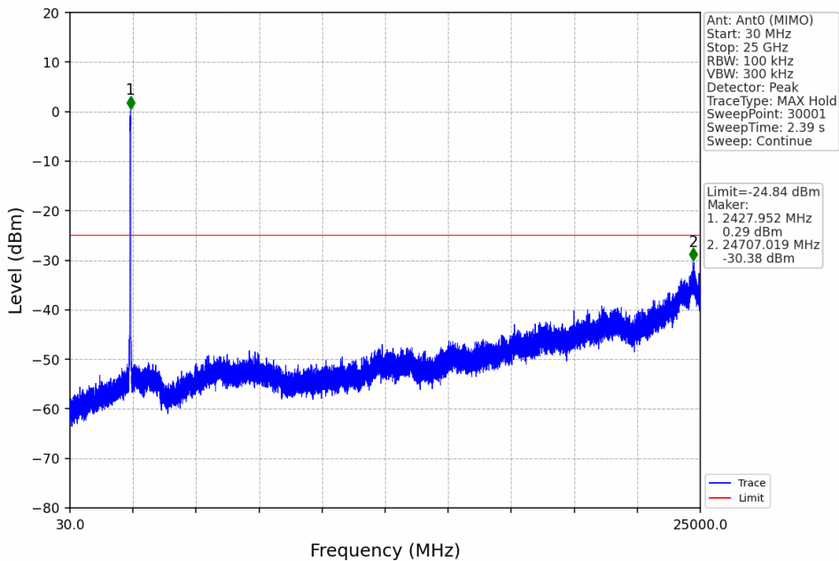
802.11ax(HEW40)_LCH_2422MHz_RU484_Left_Ant0 (MIMO)_NTNV
