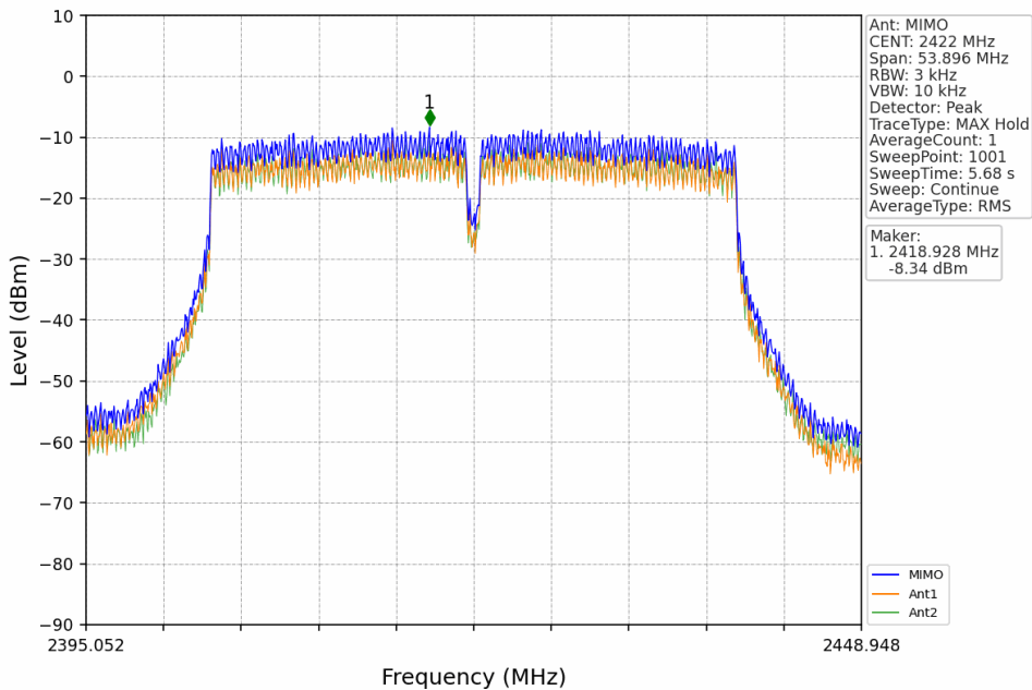
802.11n(HT40)_LCH_2422MHz_MIMO_NTNV
