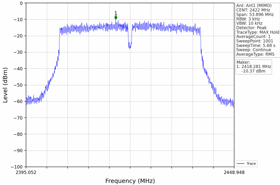
802.11n(HT40)_LCH_2422MHz_MIMO_NTNV
