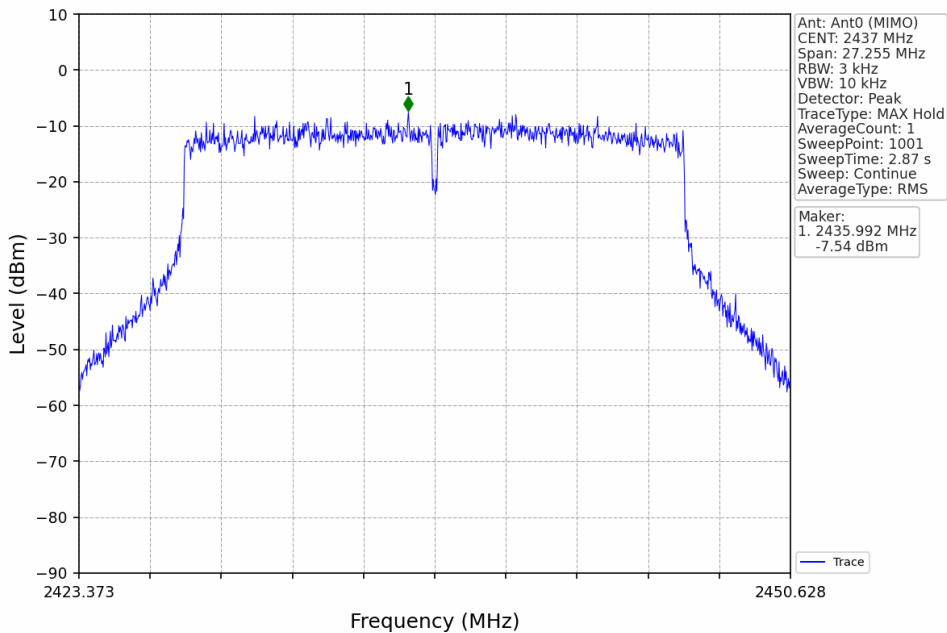
802.11ax(HEW20)_MCH_2437MHz_RU242_Left_Ant0 (MIMO)_NTNV
