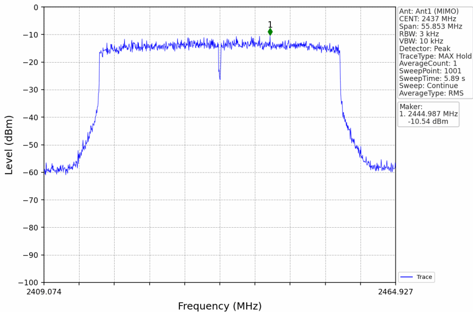
802.11ax(HEW40)_MCH_2437MHz_RU484_Left_Ant1 (MIMO)_NTNV
