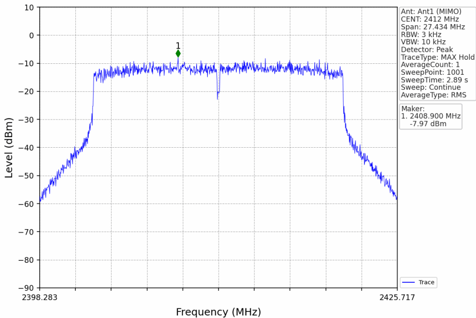
802.11ax(HEW20)_LCH_2412MHz_RU242_Left_Ant1 (MIMO)_NTNV
