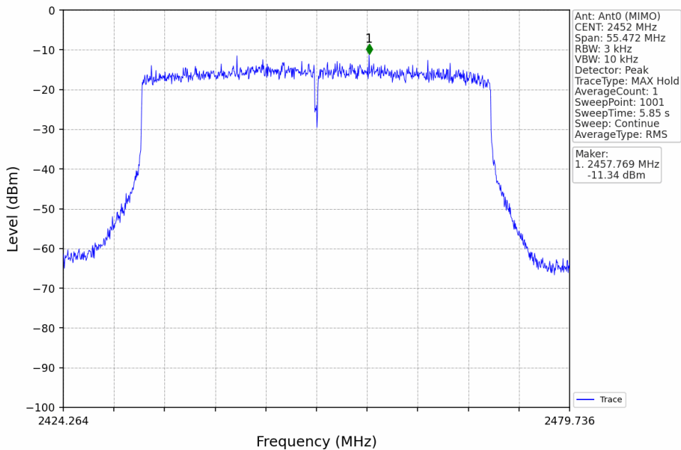
802.11ax(HEW40)_HCH_2452MHz_RU484_Left_Ant0 (MIMO)_NTNV
