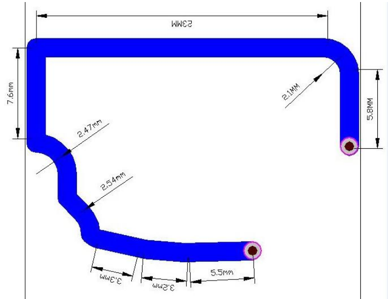
尺寸图
