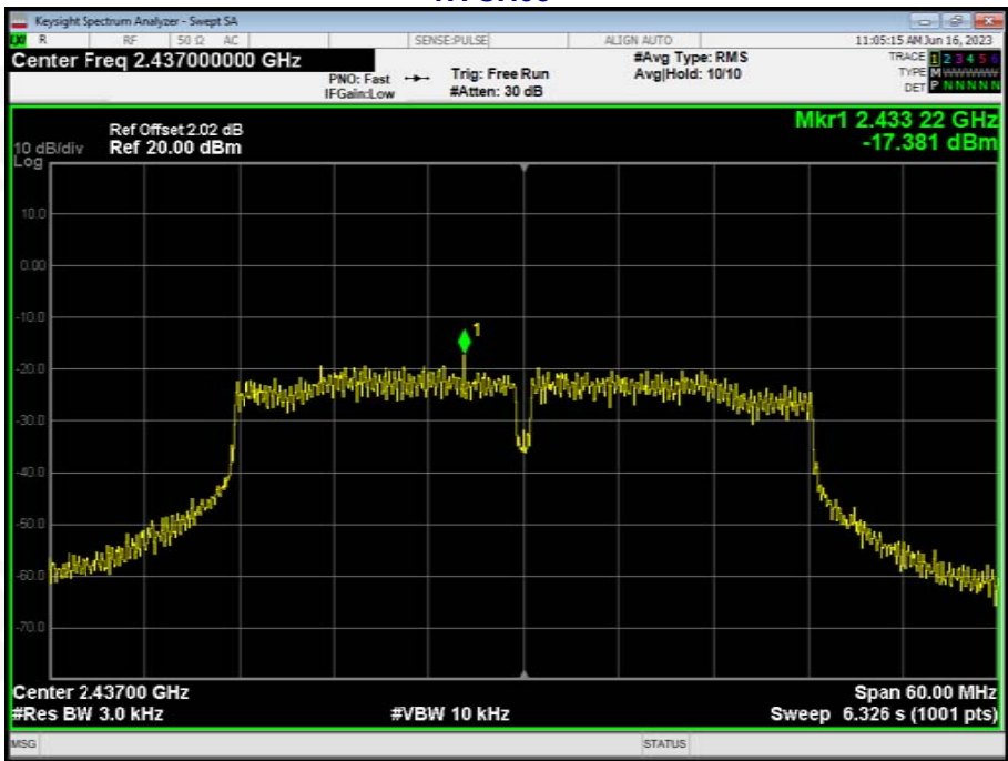
TX CH06
