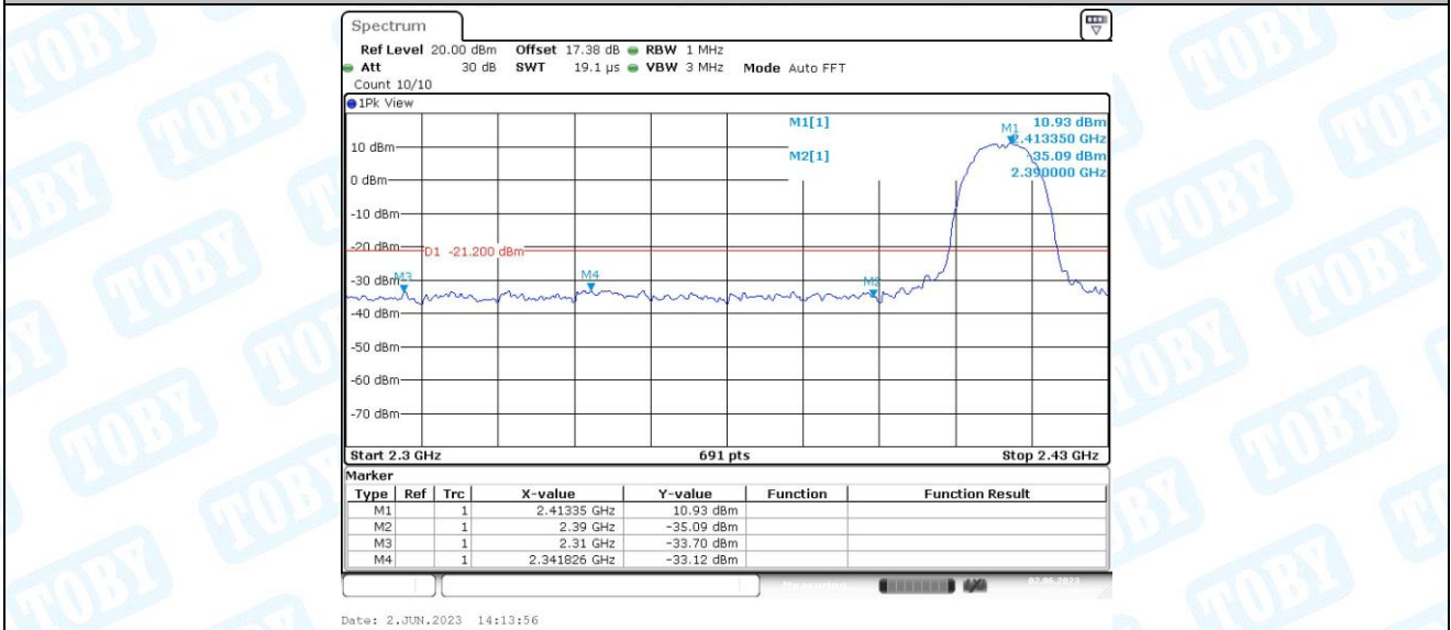
11B-CDD_Ant1_Low_2412_Peak
