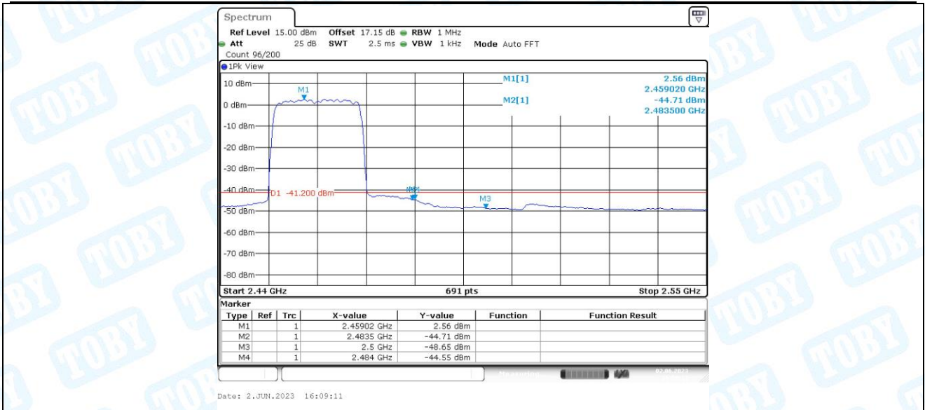
11AX20MIMO_Ant1_High_2462_AV
