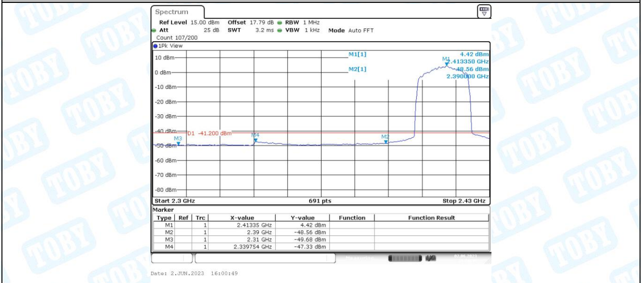
11AX20MIMO_Ant2_Low_2412_AV
