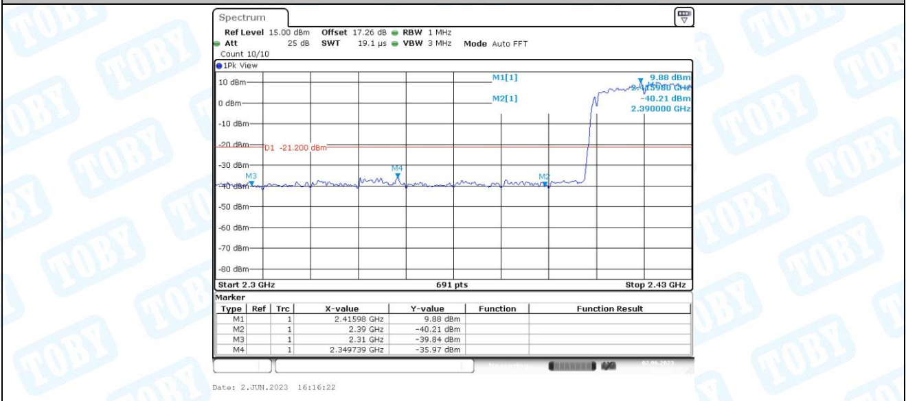
11AX40MIMO_Ant1_Low_2422_Peak
