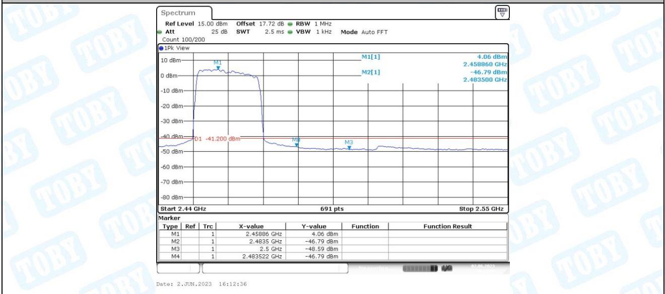
11AX20MIMO_Ant2_High_2462_AV
