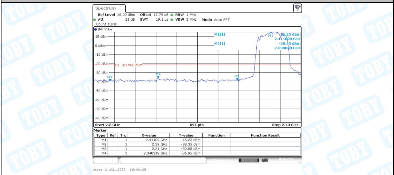
11AX20MIMO_Ant2_Low_2412_Peak
