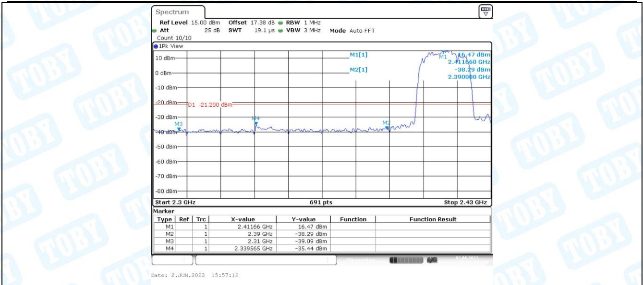
11AX20MIMO_Ant1_Low_2412_Peak
