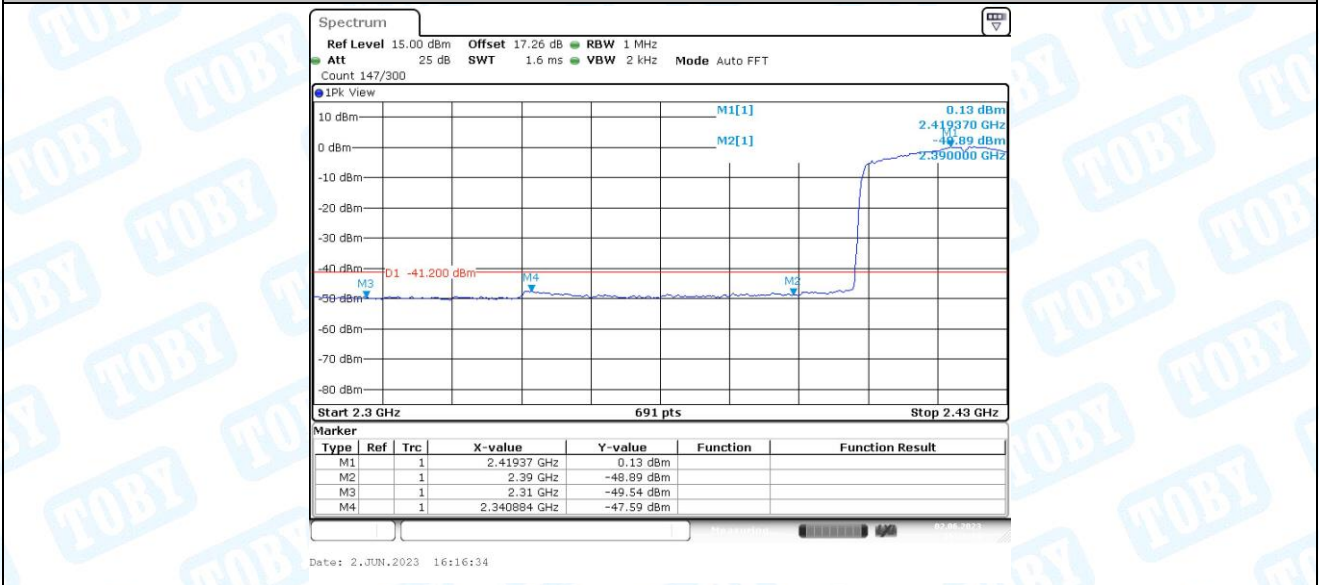
11AX40MIMO_Ant1_Low_2422_AV
