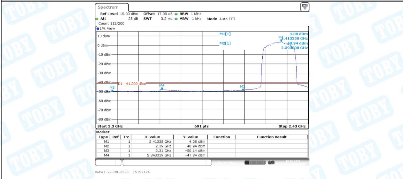
11AX20MIMO_Ant1_Low_2412_AV
