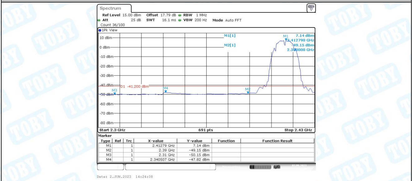
11B-CDD_Ant1_Low_2412_Peak
