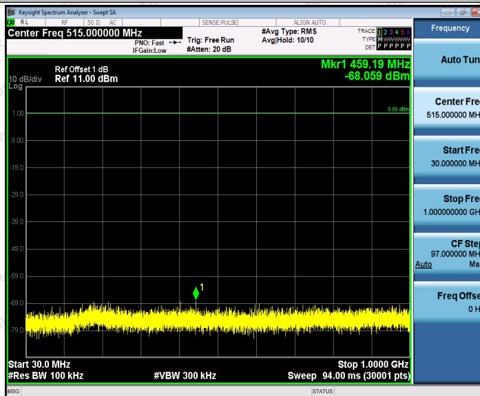
2.4G_Ant1_2438_30~1000
