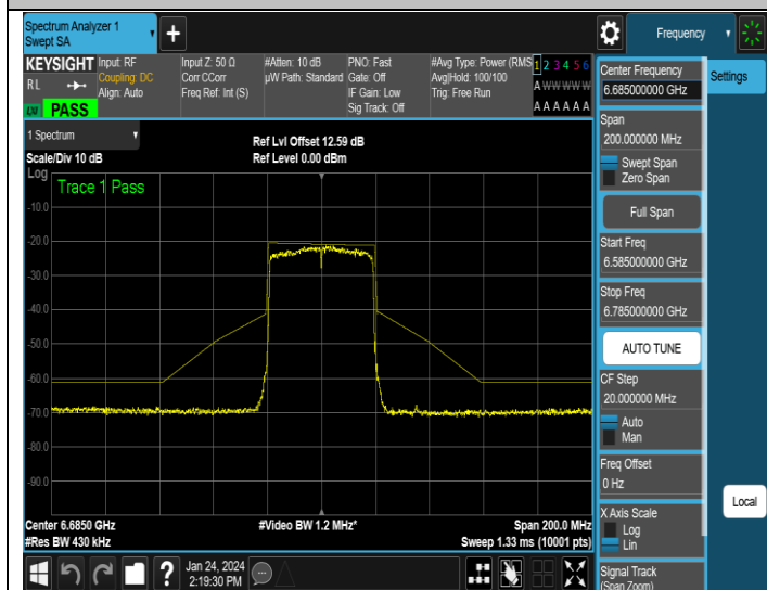
NTNV-11AX40MIMO-Ant1-6685-PASS
