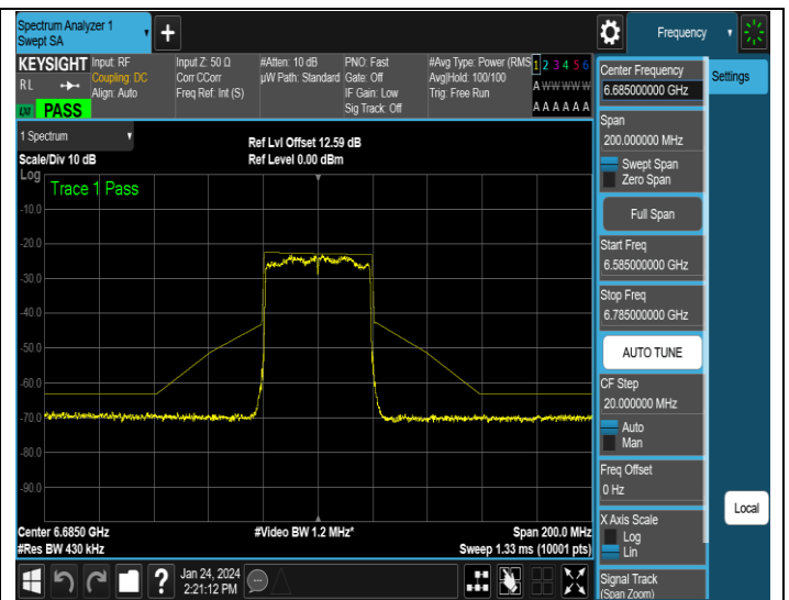
NTNV-11AX40MIMO-Ant4-6685-PASS
