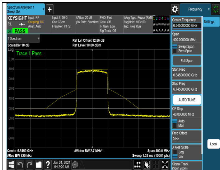
NTNV-11AX80ISO-Ant1-6545-PASS
