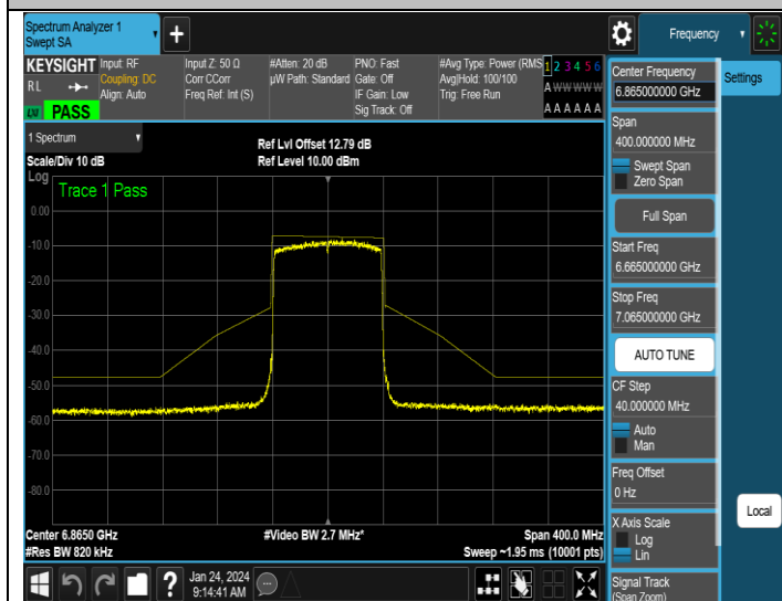
NTNV-11AX80ISO-Ant1-6865-PASS
