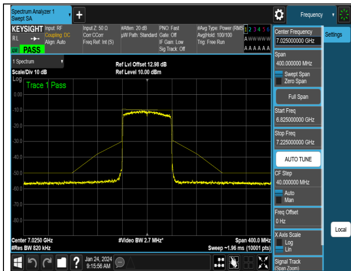
NTNV-11AX80SISO-Ant1-7025-PASS
