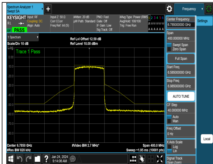
NTNV-11AX80ISO-Ant1-6785-PASS
