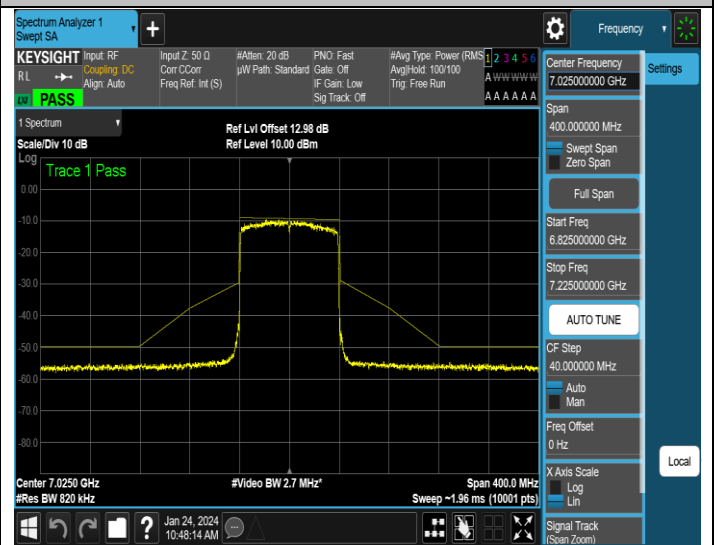
NTNV-11AX80SISO-Ant4-7025-PASS
