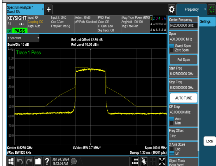
NTNV-11AX80ISO-Ant1-6625-PASS
