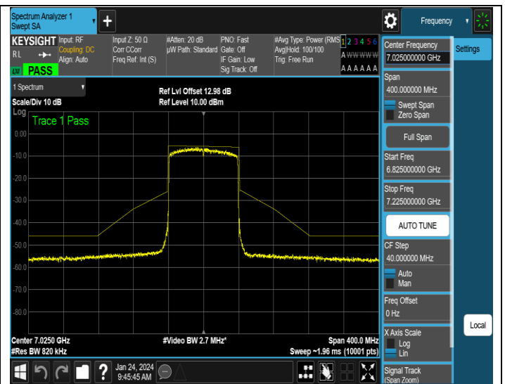
NTNV-11AX80SISO-Ant2-7025-PASS
