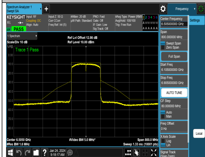
NTNV-11AX160SISO-Ant1-6505-PASS
