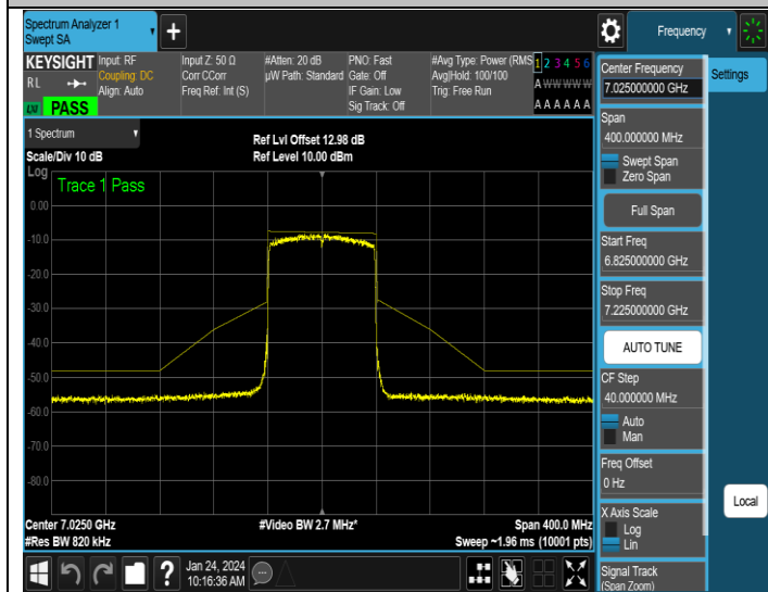
NTNV-11AX80SISO-Ant3-7025-PASS
