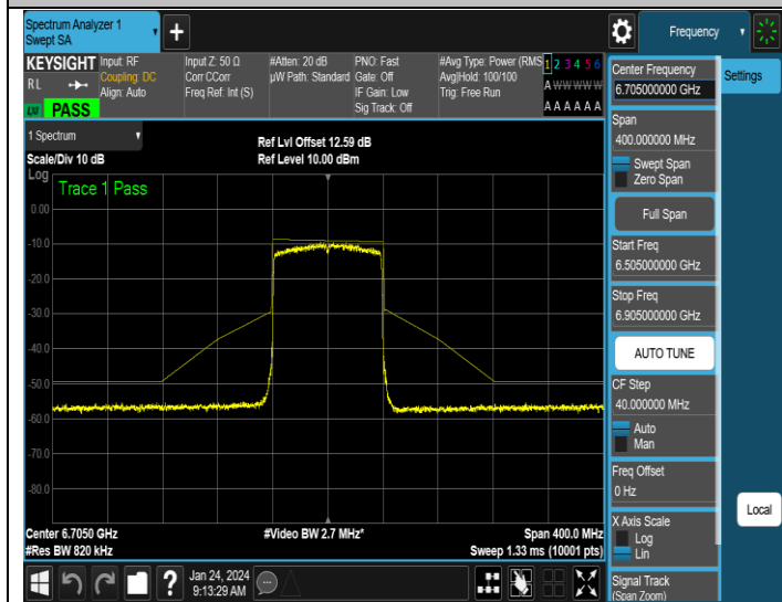
NTNV-11AX80ISO-Ant1-6705-PASS
