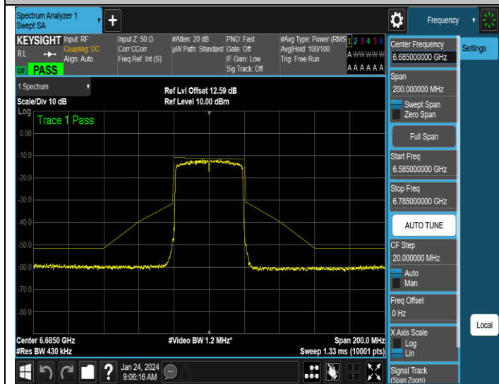
NTNV-11AX40ISO-Ant1-6685-PASS
