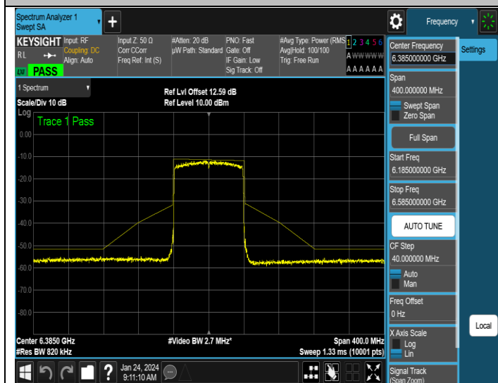
NTNV-11AX80ISO-Ant1-6385-PASS
