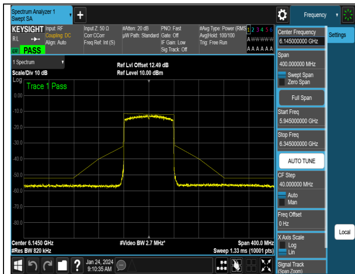
NTNV-11AX80ISO-Ant1-6145-PASS
