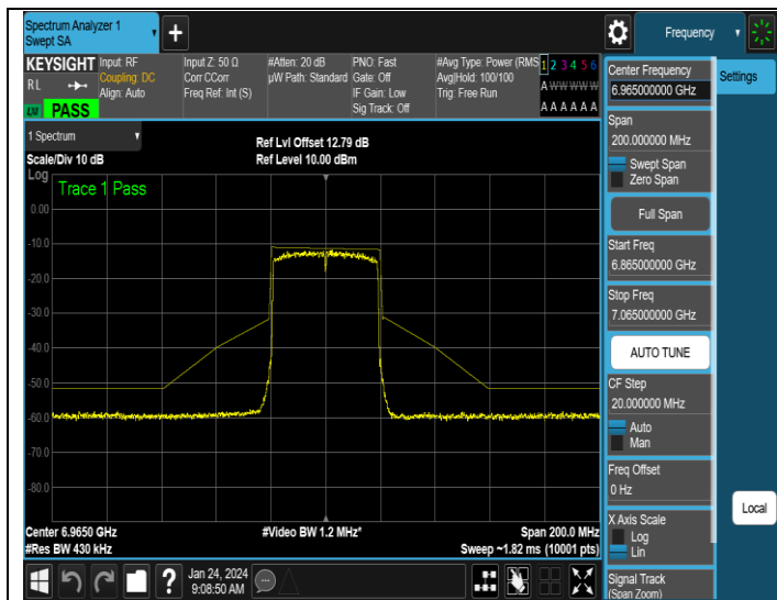
NTNV-11AX40ISO-Ant1-6965-PASS
