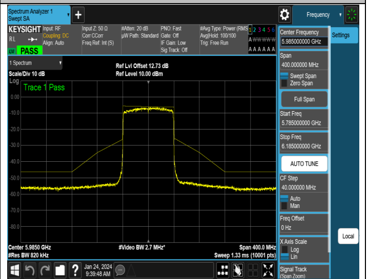
NTNV-11AX80SISO-Ant2-5985-PASS
