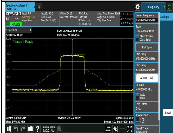
NTNV-11AX80SISO-Ant1-5985-PASS
