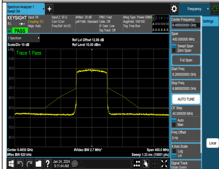
NTNV-11AX80ISO-Ant1-6465-PASS
