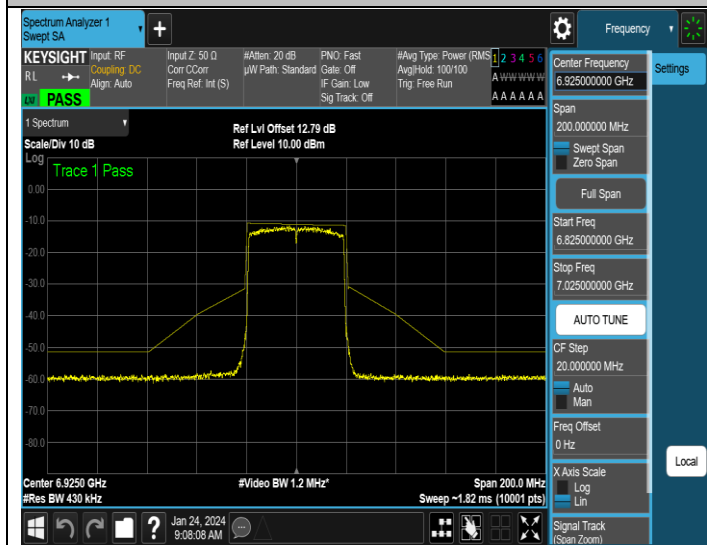
NTNV-11AX40ISO-Ant1-6925-PASS
