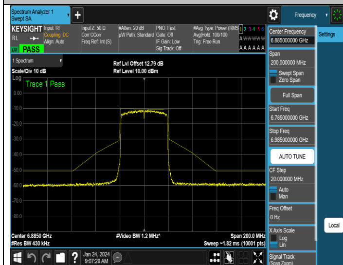
NTNV-11AX40SISO-Ant1-6885-PASS
