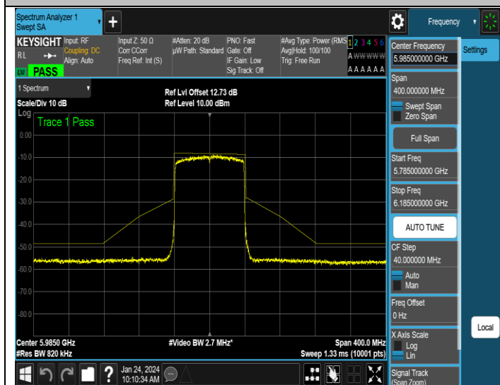
NTNV-11AX80SISO-Ant3-5985-PASS
