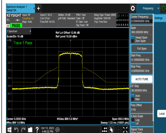
NTNV-11AX160SISO-Ant1-6505-PASS
