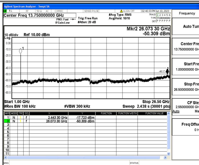
11N40MIMO_Ant2_2452_0~Reference
