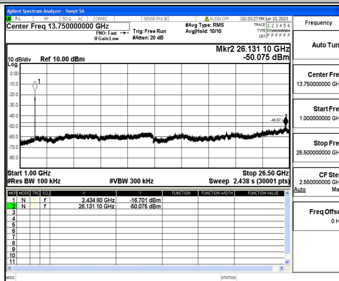
11N40MIMO_Ant2_2437_0~Reference
