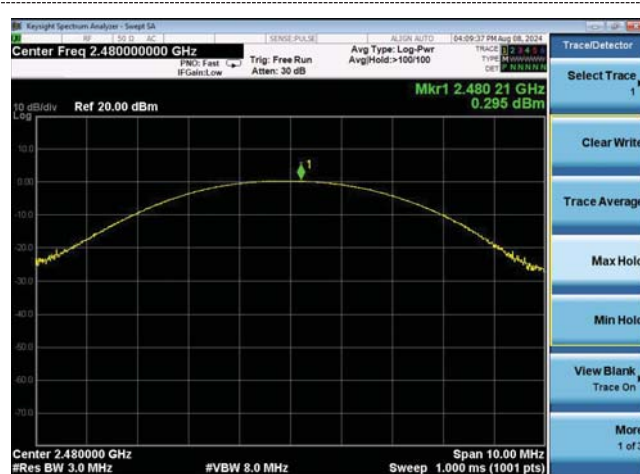
GFSK(CH78)
