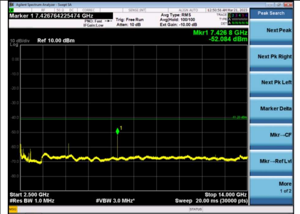
2.5-14 GHz Ch 25
