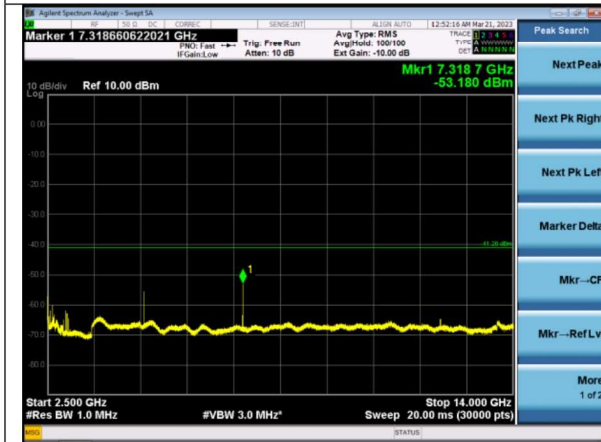
2.5-14 GHz Ch 18
