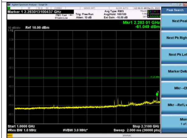
1-2.31 GHz Ch 25
