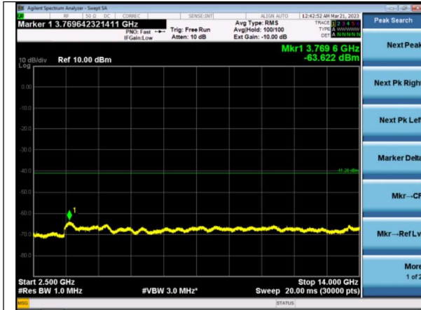
2.5-14 GHz Ch 26
