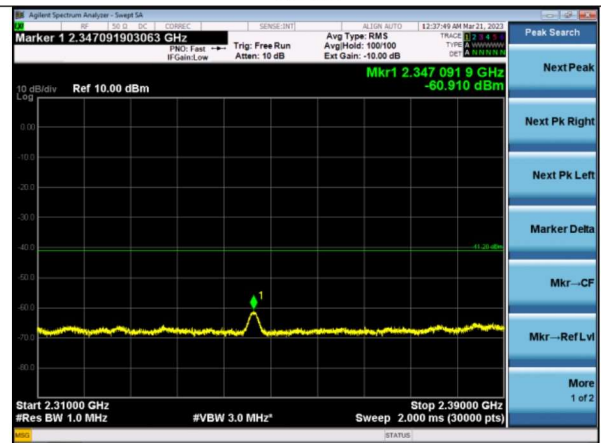
2.31-2.39 GHz Ch 25
