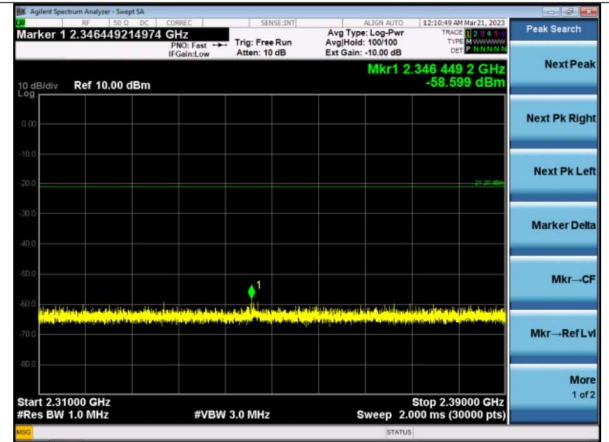
2.31-2.39 GHz Ch 26
