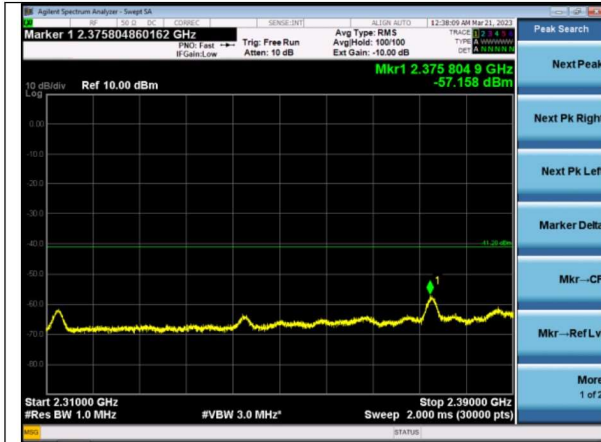
2.31-2.39 GHz Ch 18
