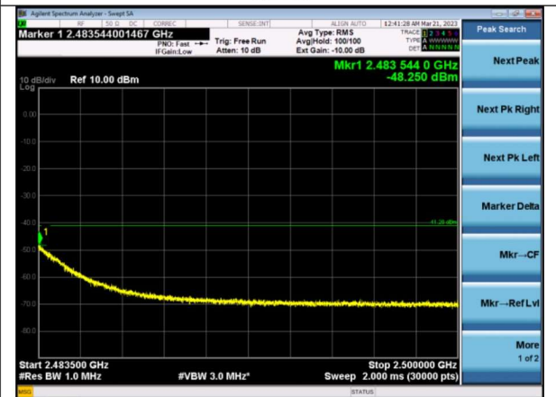
2.4835-2.5 GHz Ch 26
