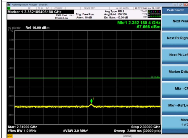
2.31-2.39 GHz Ch 26
