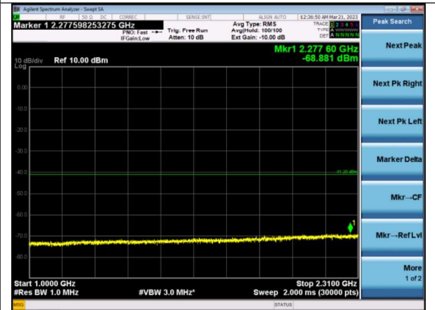
1-2.31 GHz Ch 26
