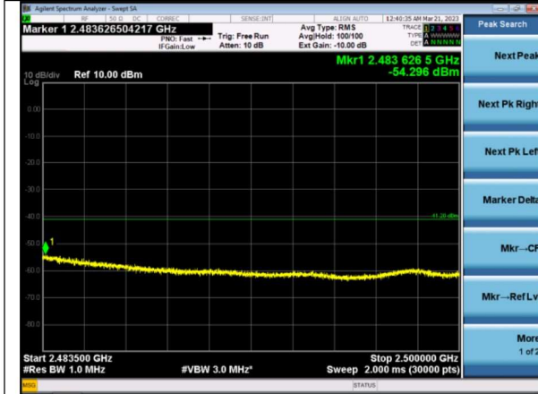
2.4835-2.5 GHz Ch 25
