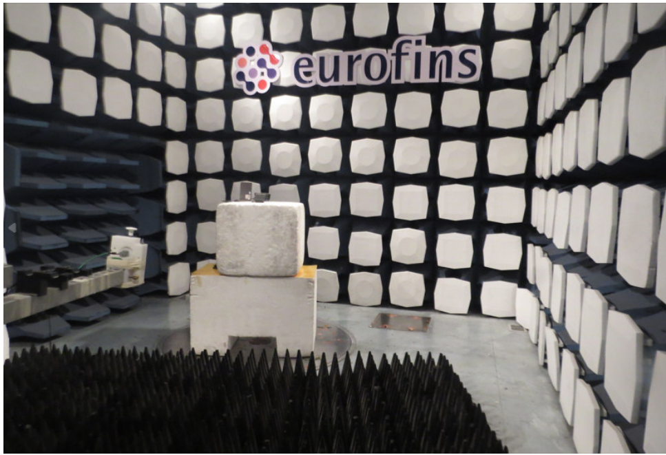
1GHz-18GHz
