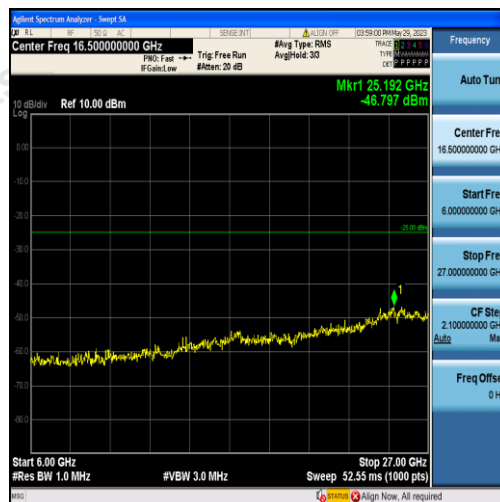
Band7-10MHz-QPSK-21400-50RB#0-Range3:6000~27000MHz
