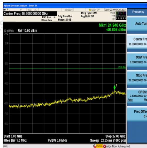
Band7-10MHz-16QAM-21400-50RB#0-Range3:6000~27000MHz
