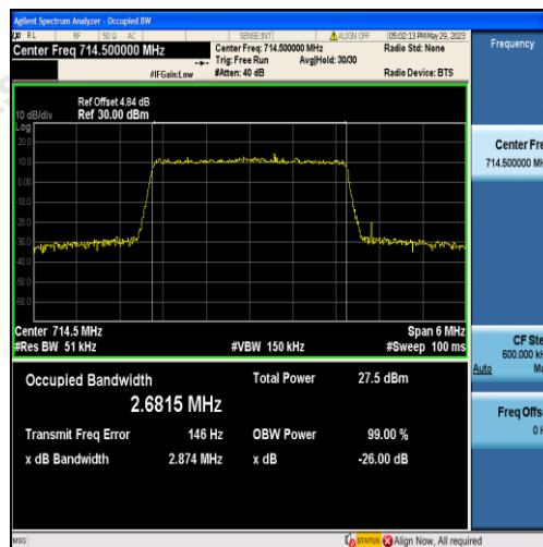
Band12-3MHz-QPSK-23165-15RB#0-2.6815
