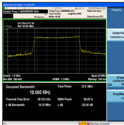
Band2-20MHz-16QAM-19100-100RB#0-18.060
