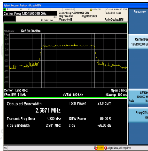
Band2-3MHz-QPSK-18615-15RB#0-2.6871
