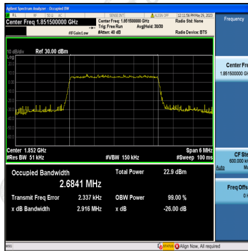
Band2-3MHz-16QAM-18615-15RB#0-2.6841
