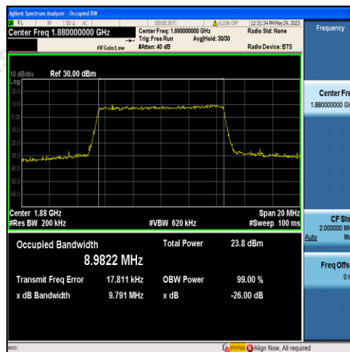
Band2-10MHz-QPSK-18900-50RB#0-8.9822
