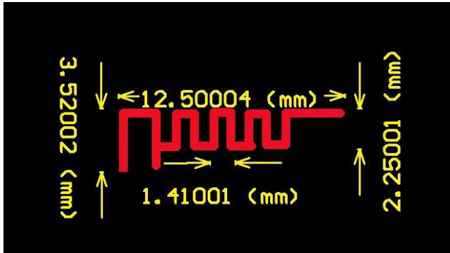
Antenna Photo & Length (mm) 天线照片和长度 (mm)
