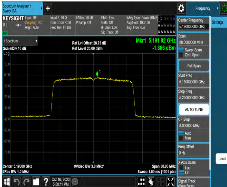
11AX40MIMO_Ant2_5190
