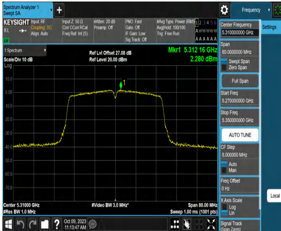
11AC40MIMO_Ant2_5310
