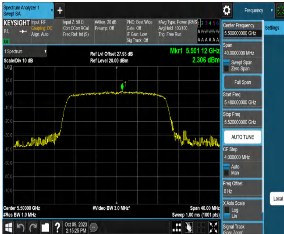
11AX20MIMO_Ant2_5500
