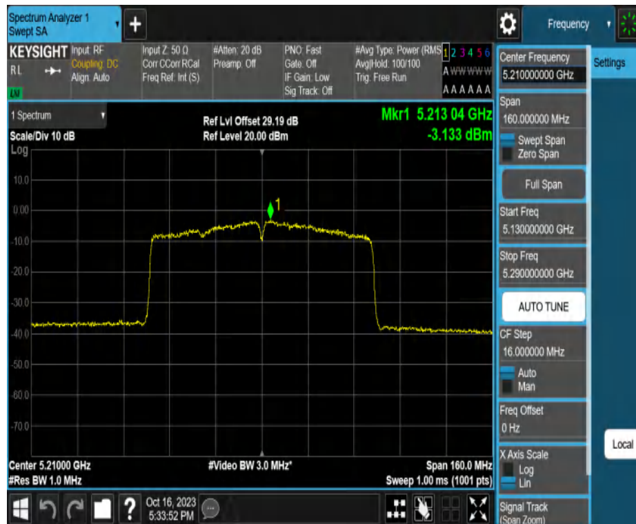
11AC80MIMO_Ant2_5210
