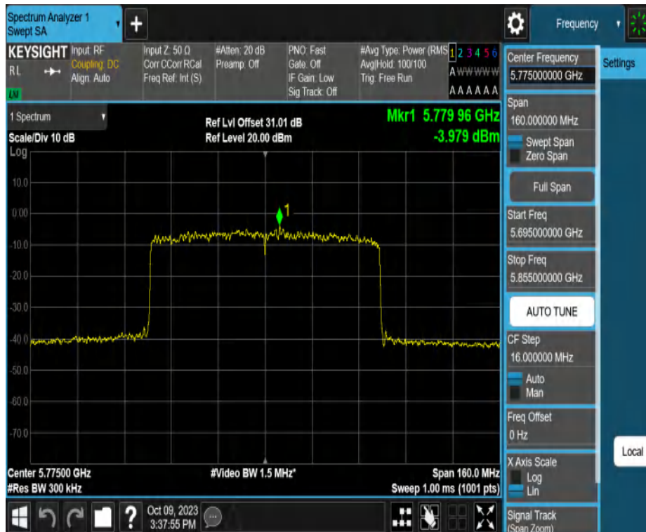
11AX80MIMO_Ant2_5775
