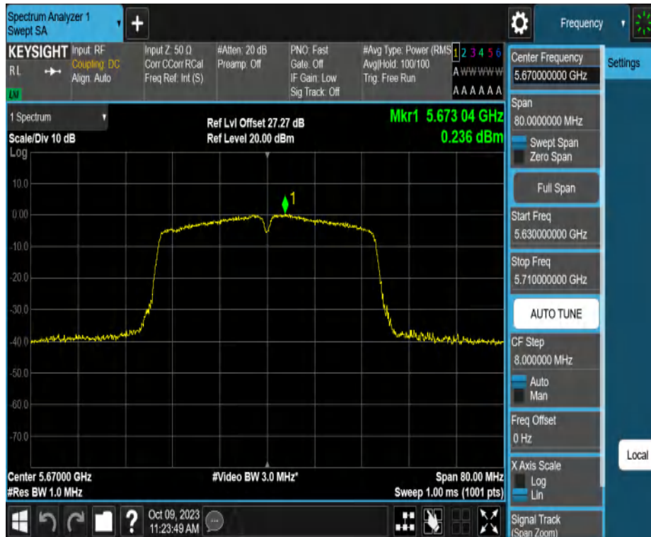
11AC40MIMO_Ant2_5670
