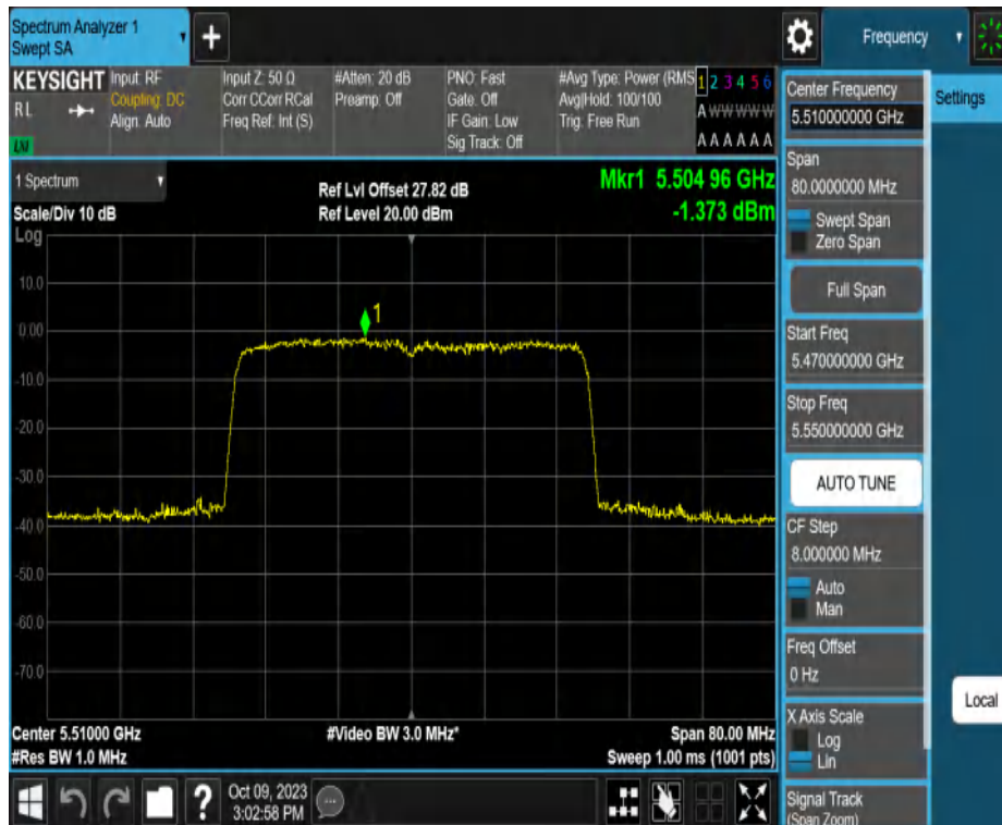
11AX40MIMO_Ant2_5510
