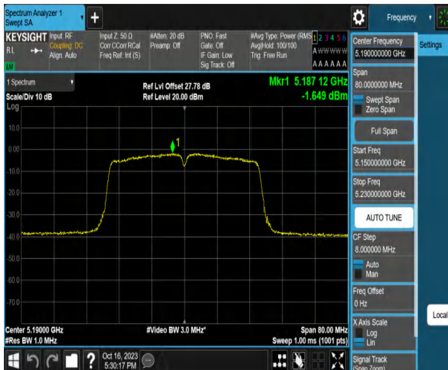
11AC40MIMO_Ant2_5190
