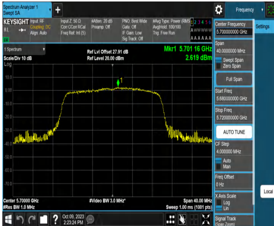
11AX20MIMO_Ant2_5700
