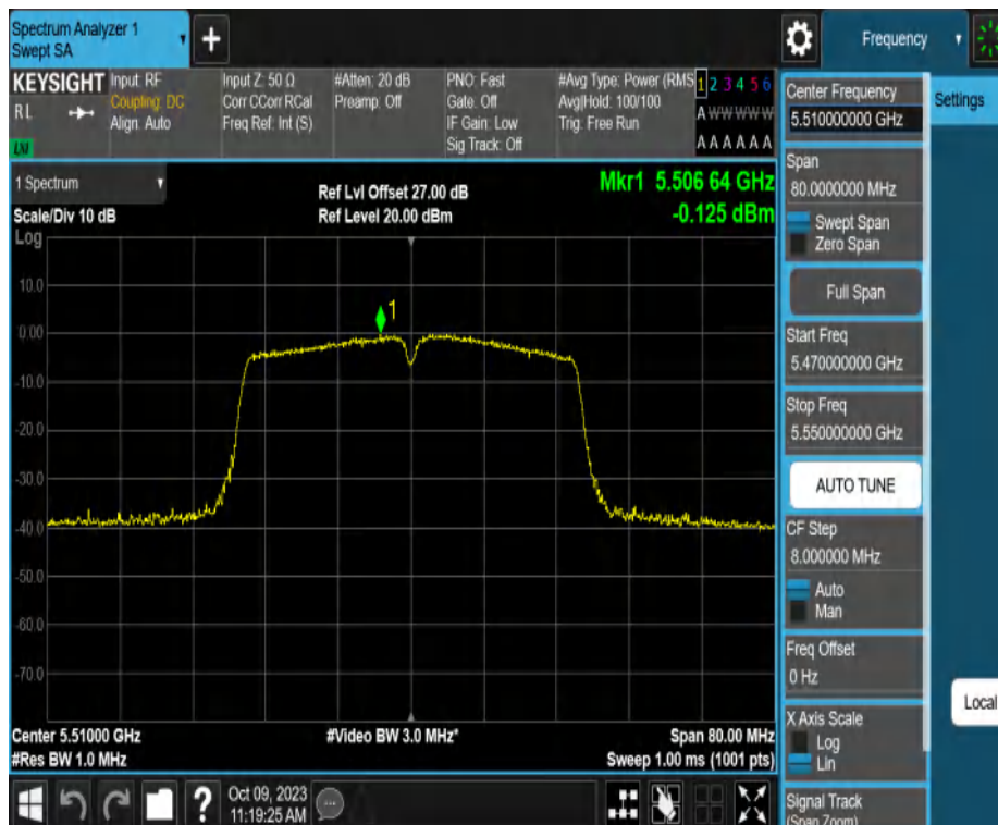
11AC40MIMO_Ant2_5510
