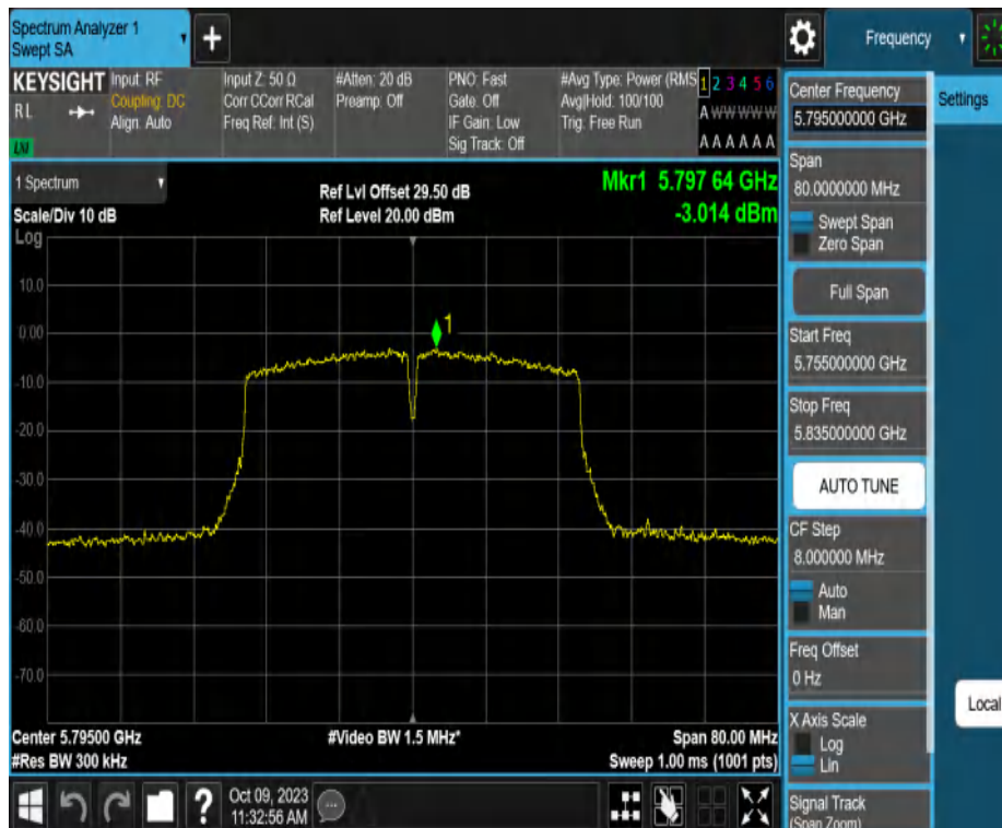
11AC40MIMO_Ant2_5795
