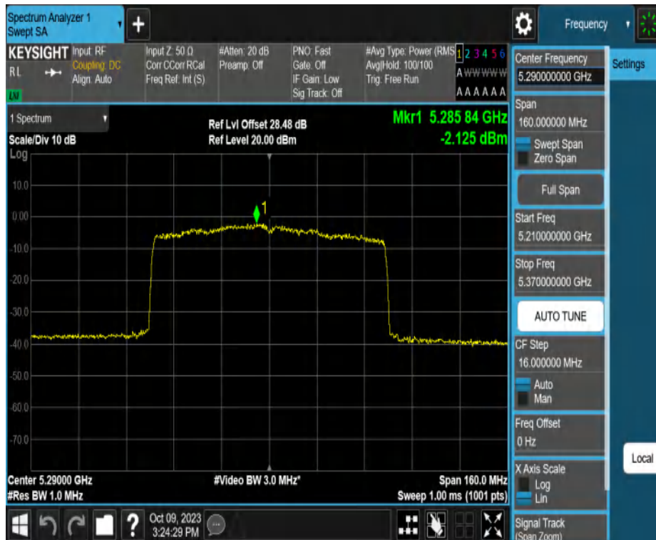
11AX80MIMO_Ant2_5290
