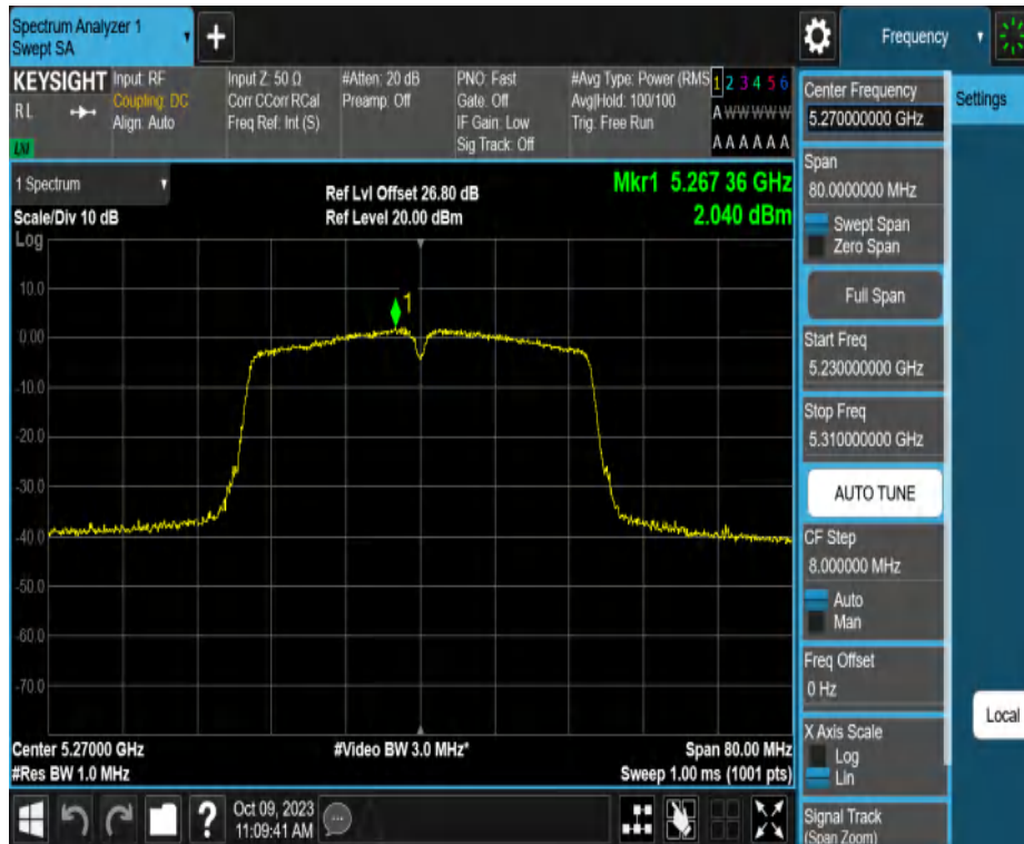
11AC40MIMO_Ant2_5270
