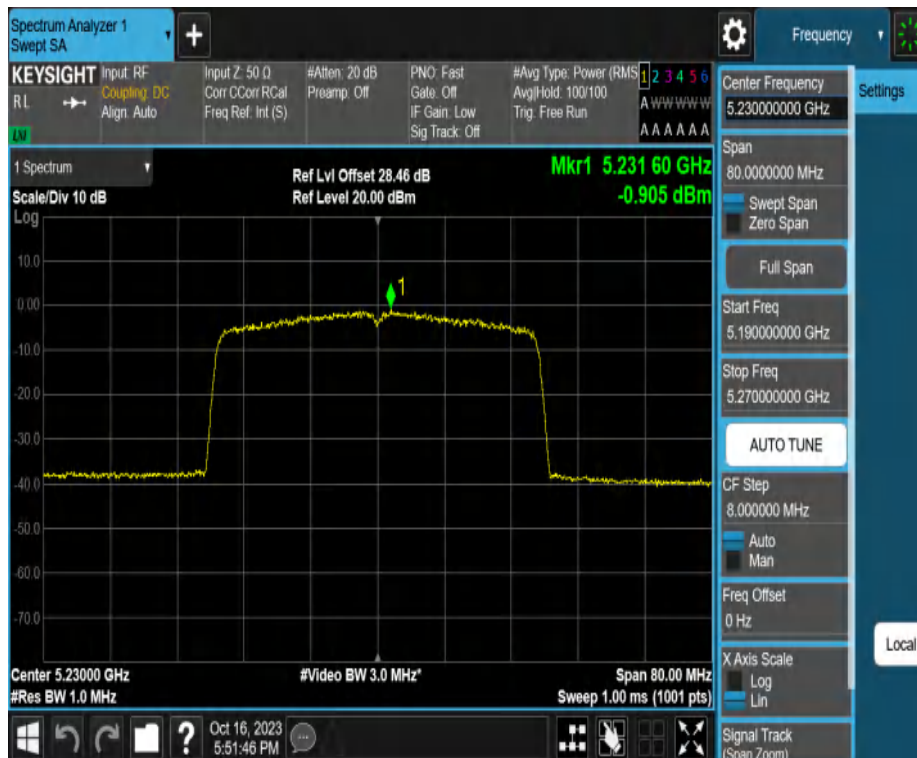
11AX40MIMO_Ant2_5230
