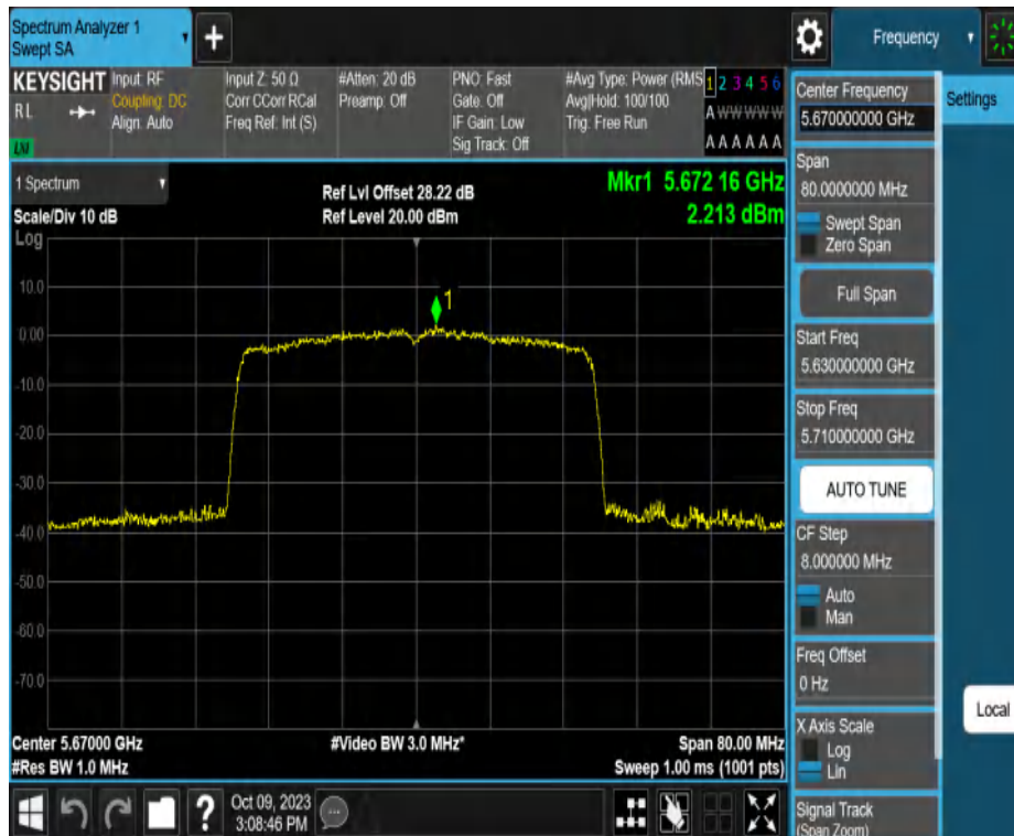
11AX40MIMO_Ant2_5670
