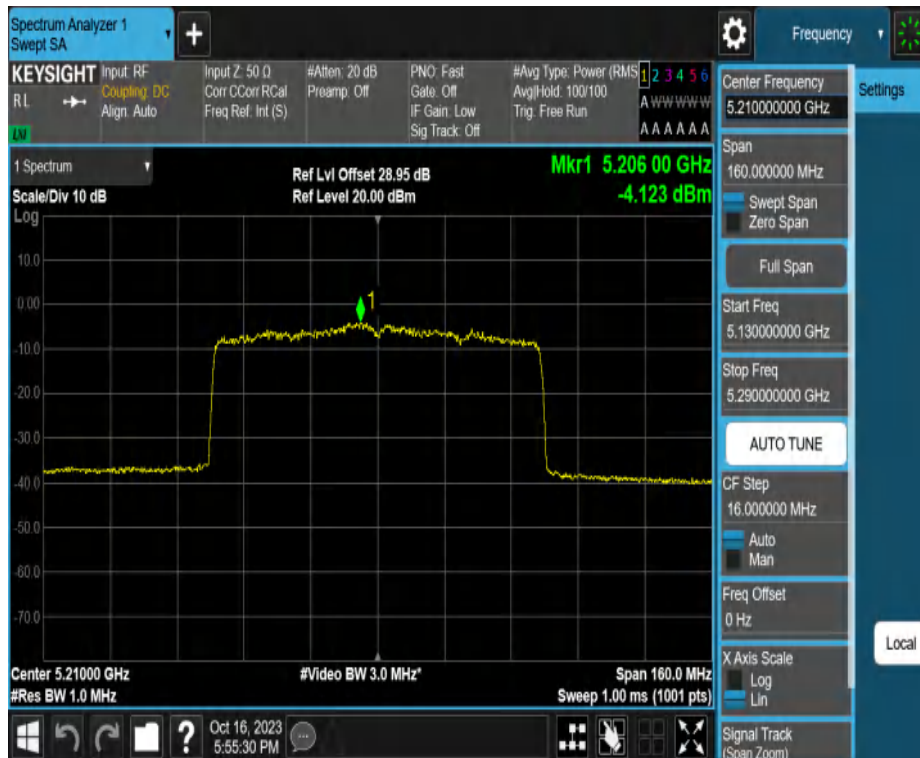
11AX80MIMO_Ant2_5210
