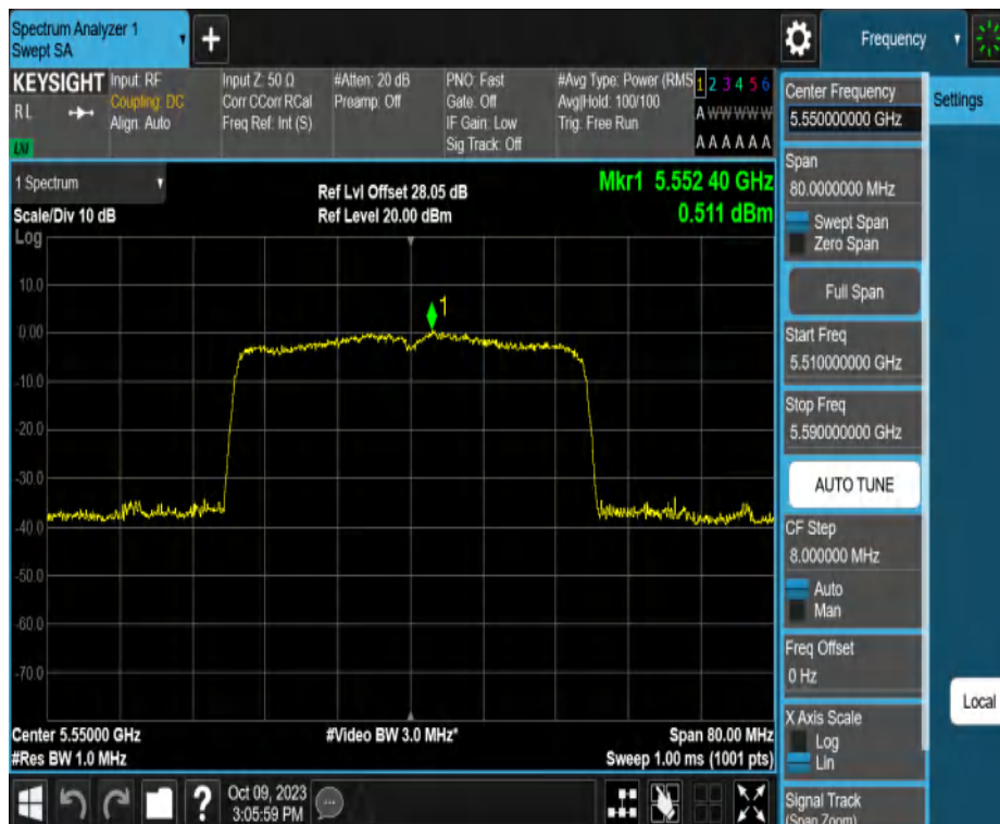
11AX40MIMO_Ant2_5550
