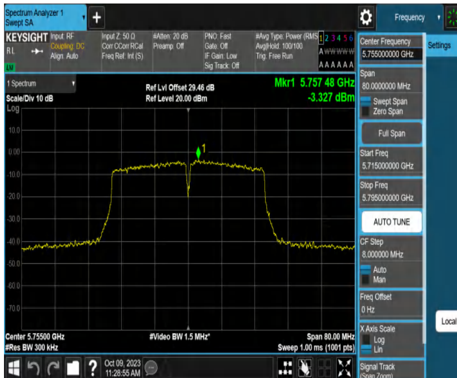
11AC40MIMO_Ant2_5755
