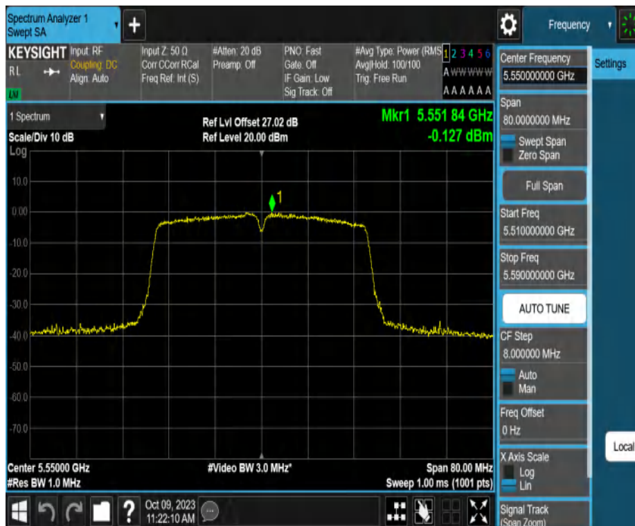
11AC40MIMO_Ant2_5550
