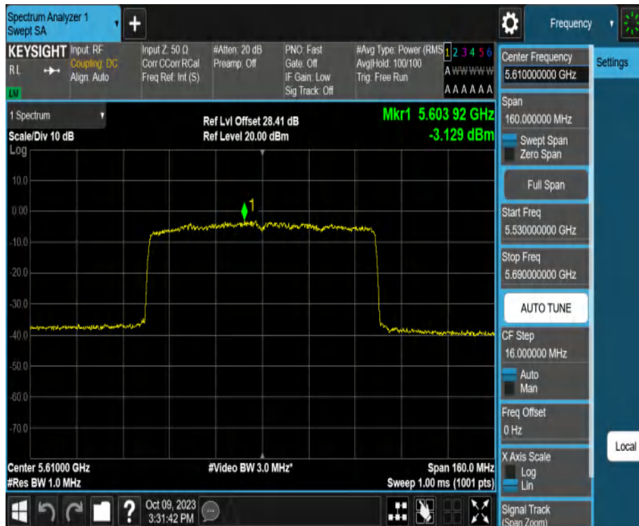
11AX80MIMO_Ant2_5610
