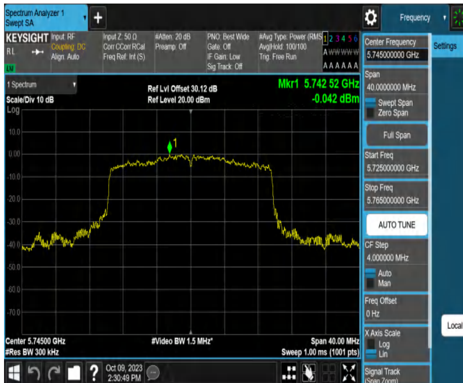
11AX20MIMO_Ant2_5745
