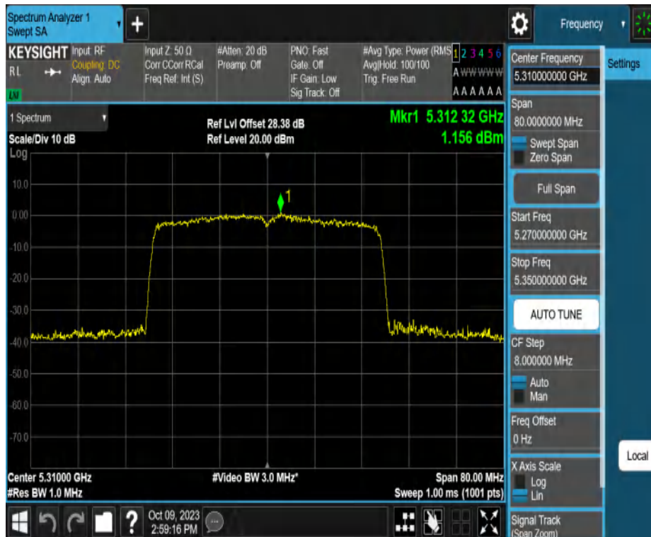
11AX40MIMO_Ant2_5310
