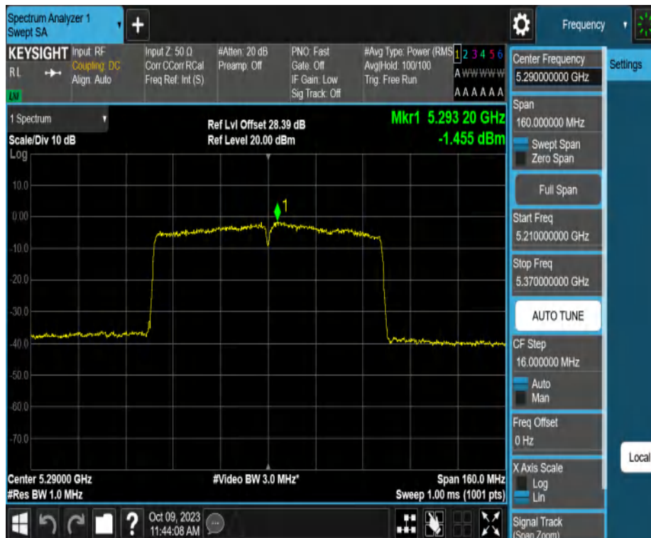
11AC80MIMO_Ant2_5290
