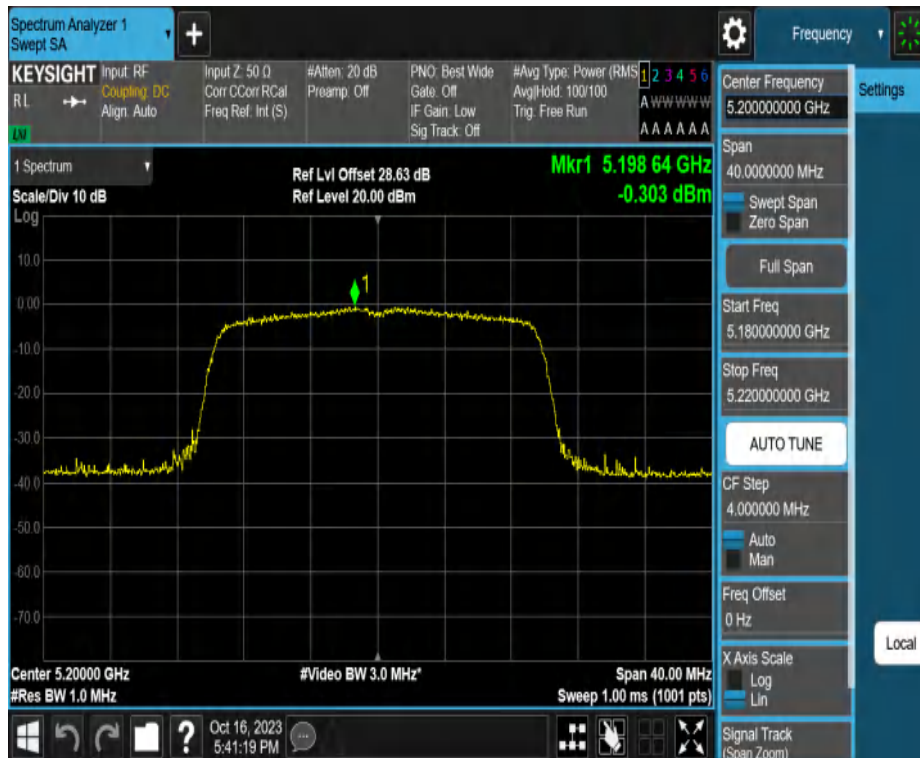
11AX20MIMO_Ant2_5200
