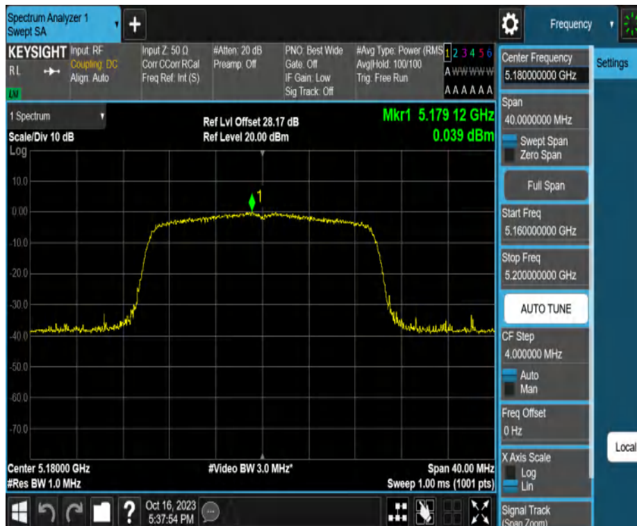
11AX20MIMO_Ant2_5180
