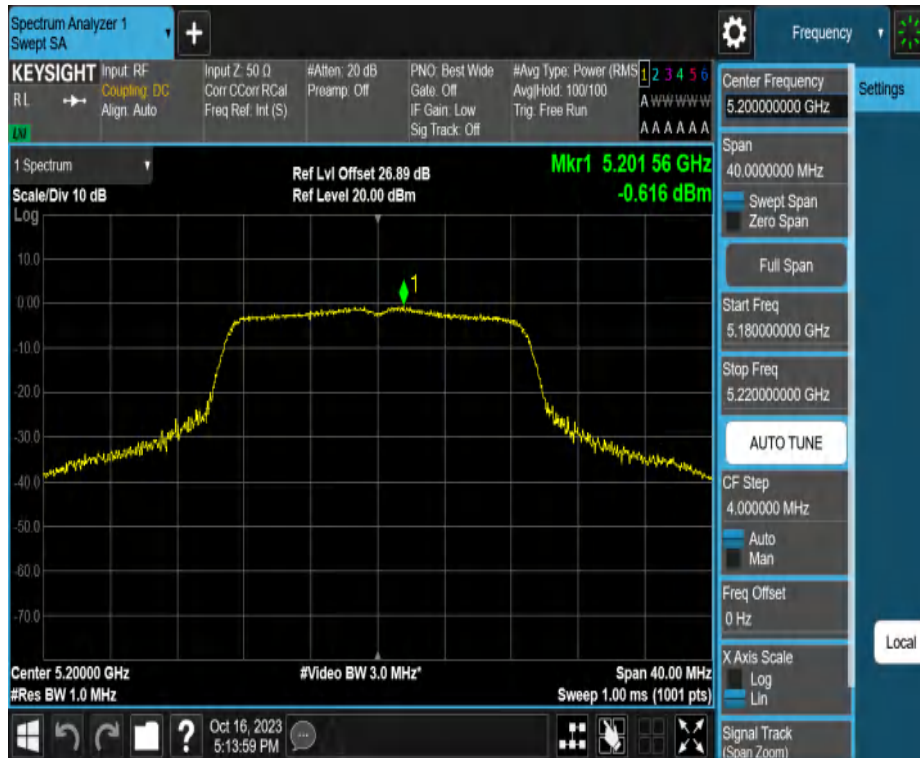
11AC20MIMO_Ant2_5200
