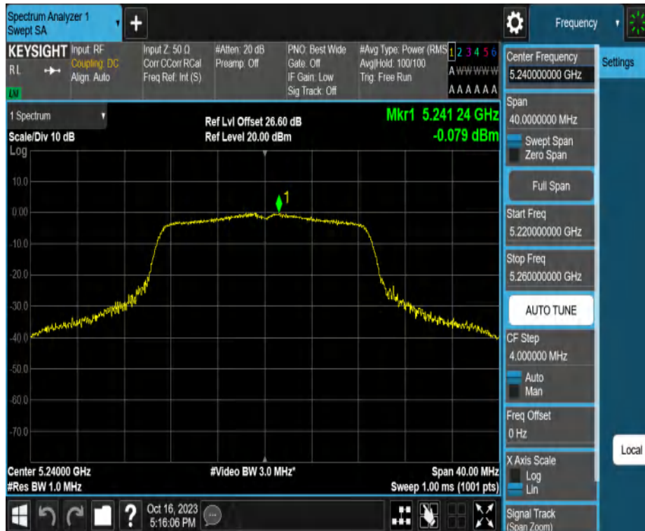
11AC20MIMO_Ant2_5240
