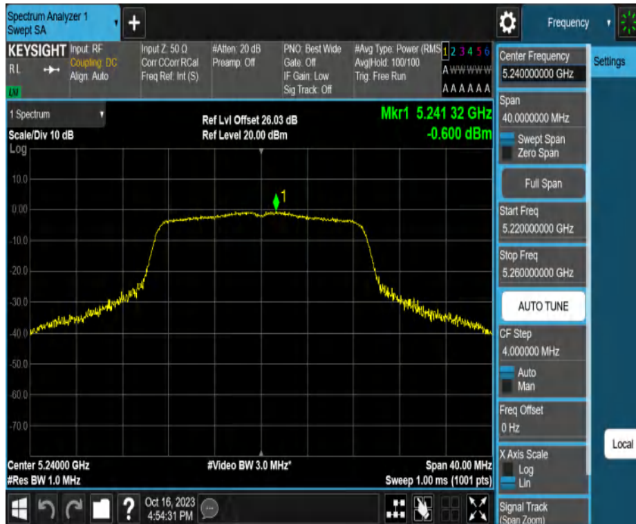
11N20MIMO_Ant2_5240
