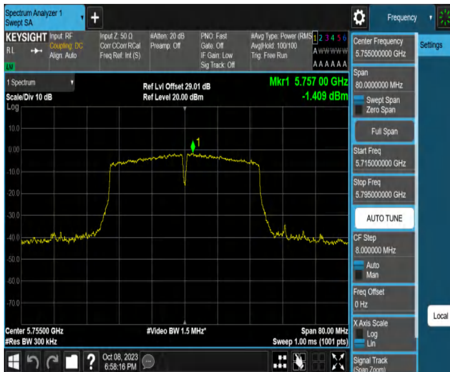
11N40MIMO_Ant2_5755
