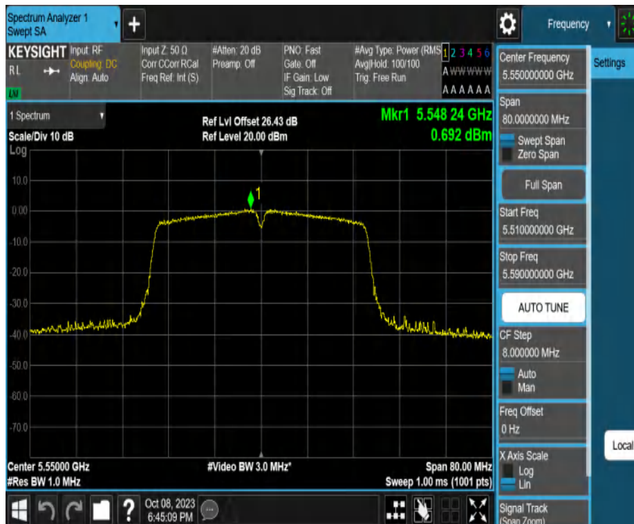
11N40MIMO_Ant2_5550
