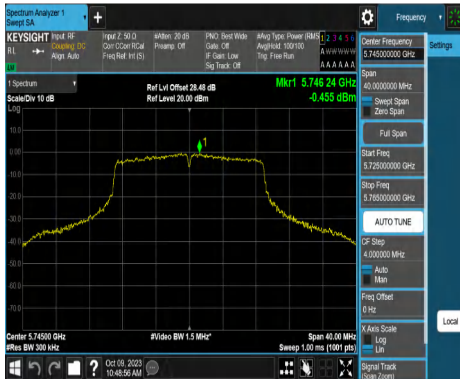
11AC20MIMO_Ant2_5745
