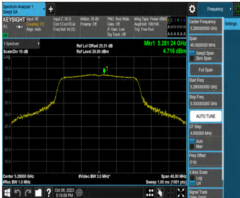
11N20MIMO_Ant2_5280
