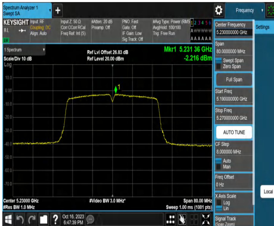
11N40MIMO_Ant2_5230
