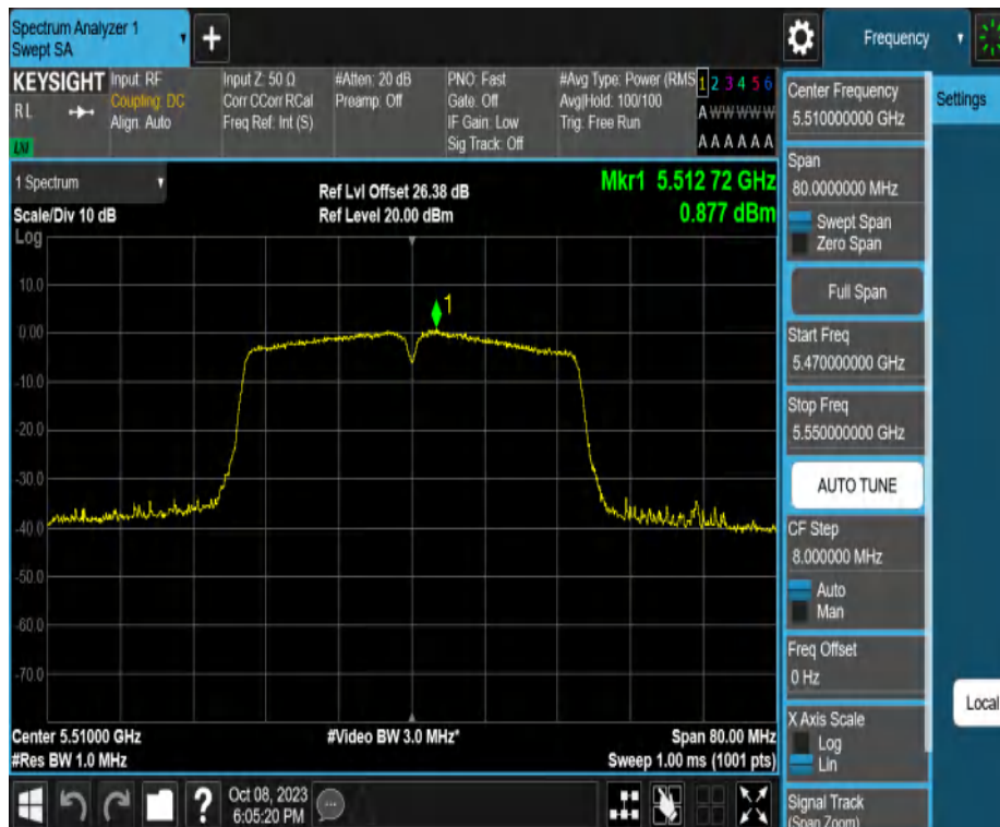
11N40MIMO_Ant2_5510
