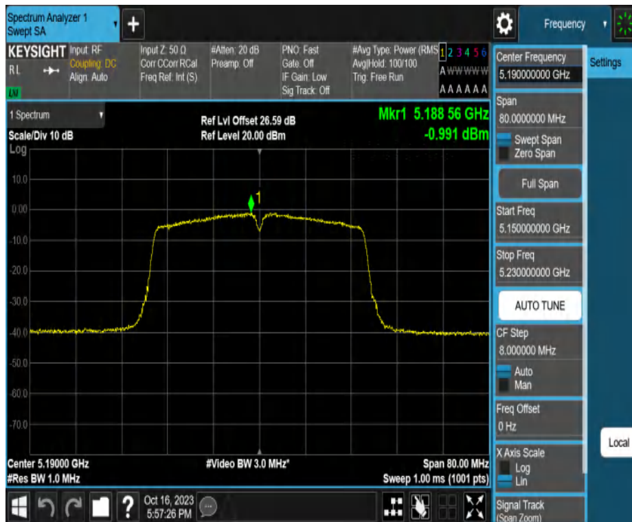
11N40MIMO_Ant2_5190
