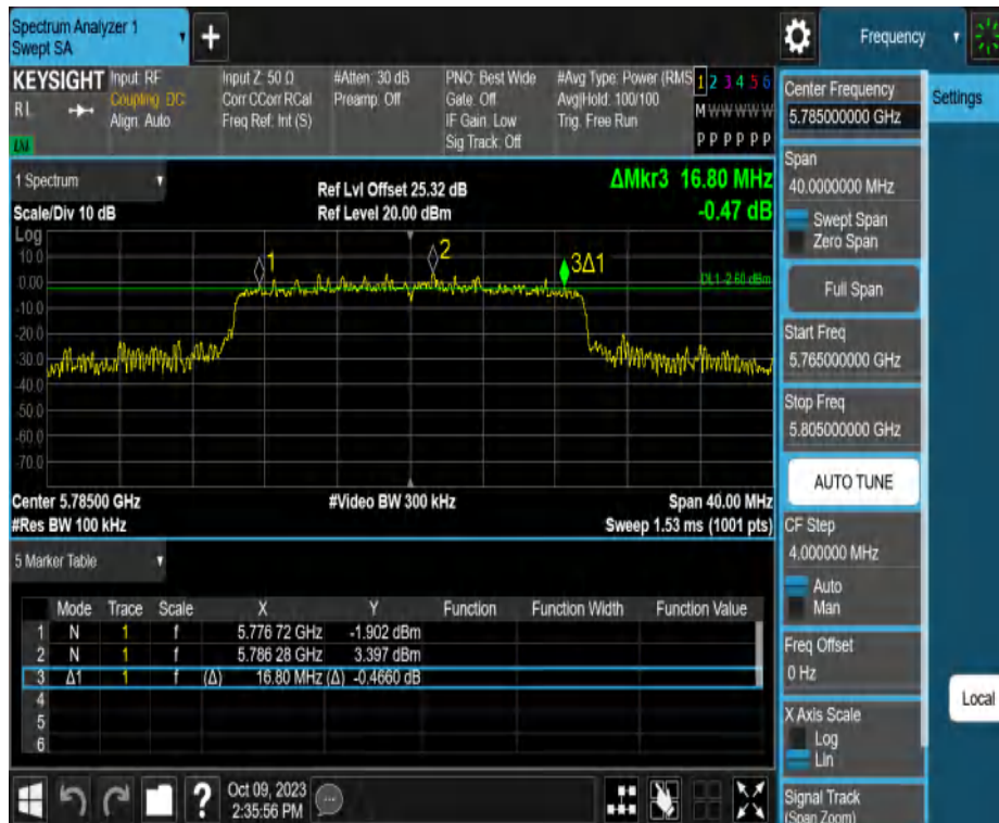
11AX20MIMO_Ant2_5785
