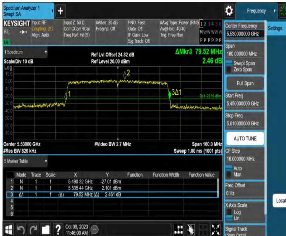
11AC80MIMO_Ant2_5530
