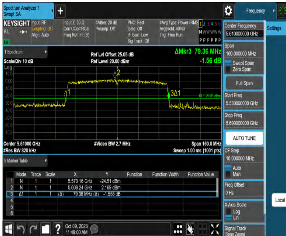
11AC80MIMO_Ant2_5610
