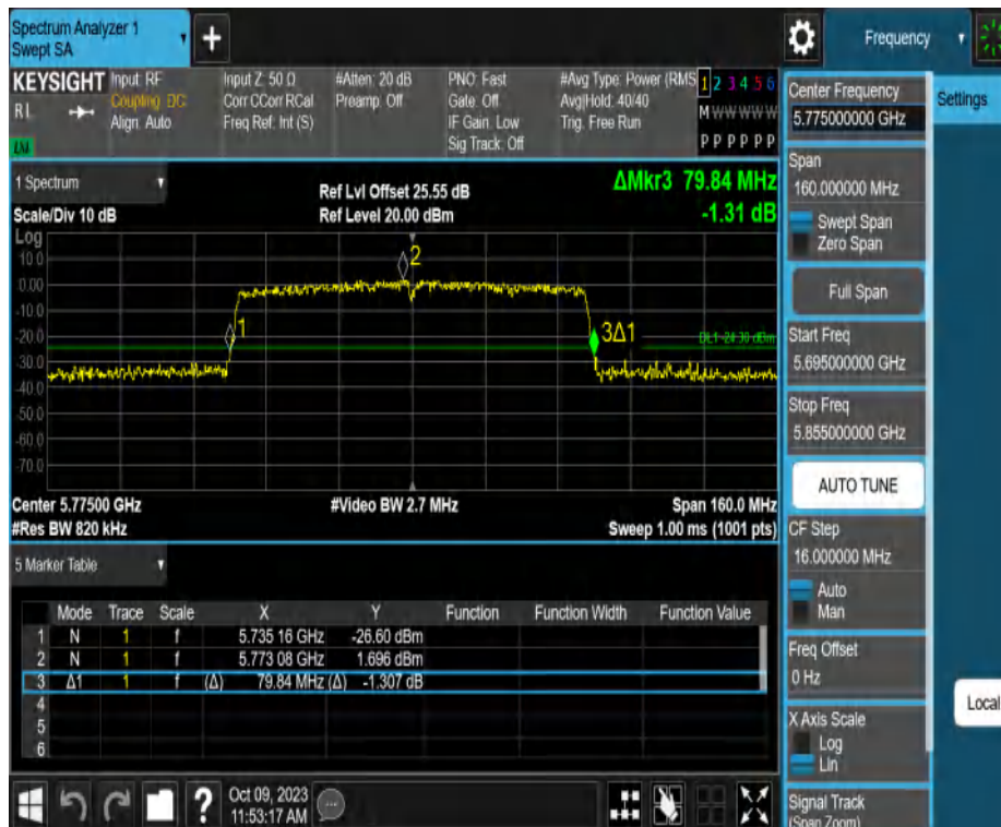
11AC80MIMO_Ant2_5775
