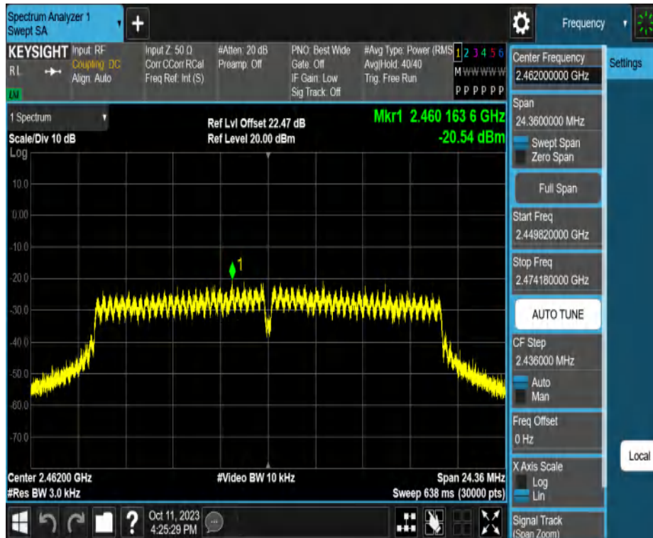
11N20MIMO_Ant2_2462
