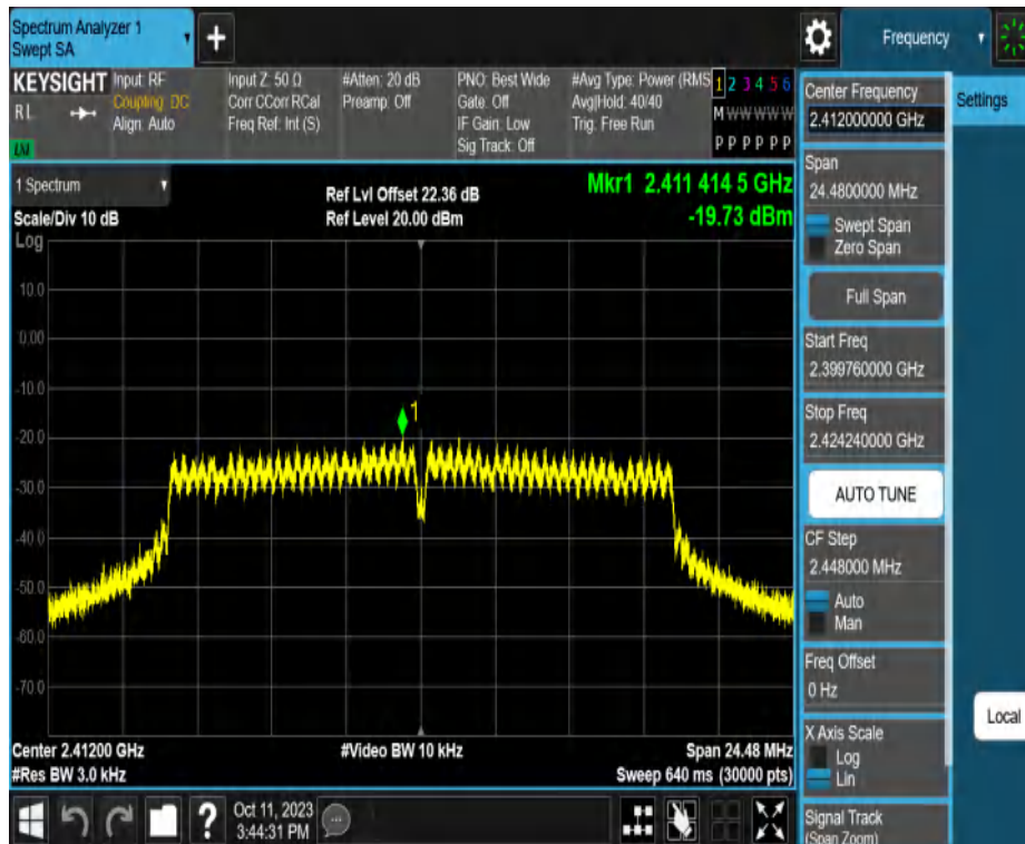
11G-CDD_Ant2_2412
