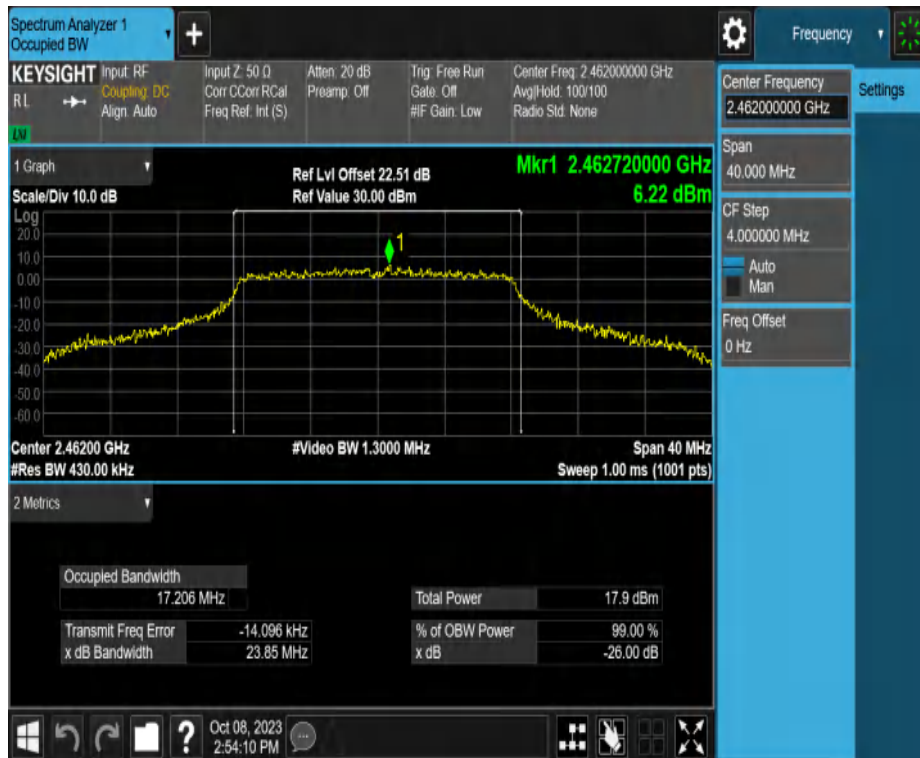
11G-CDD_Ant2_2462
