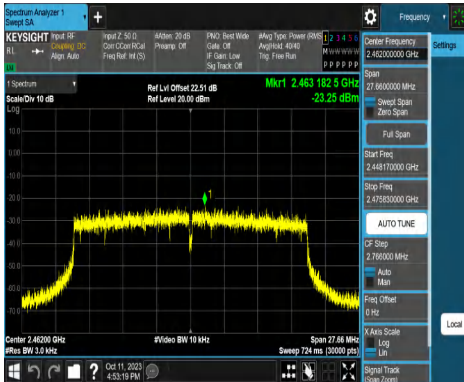
11AX20MIMO_Ant2_2462
