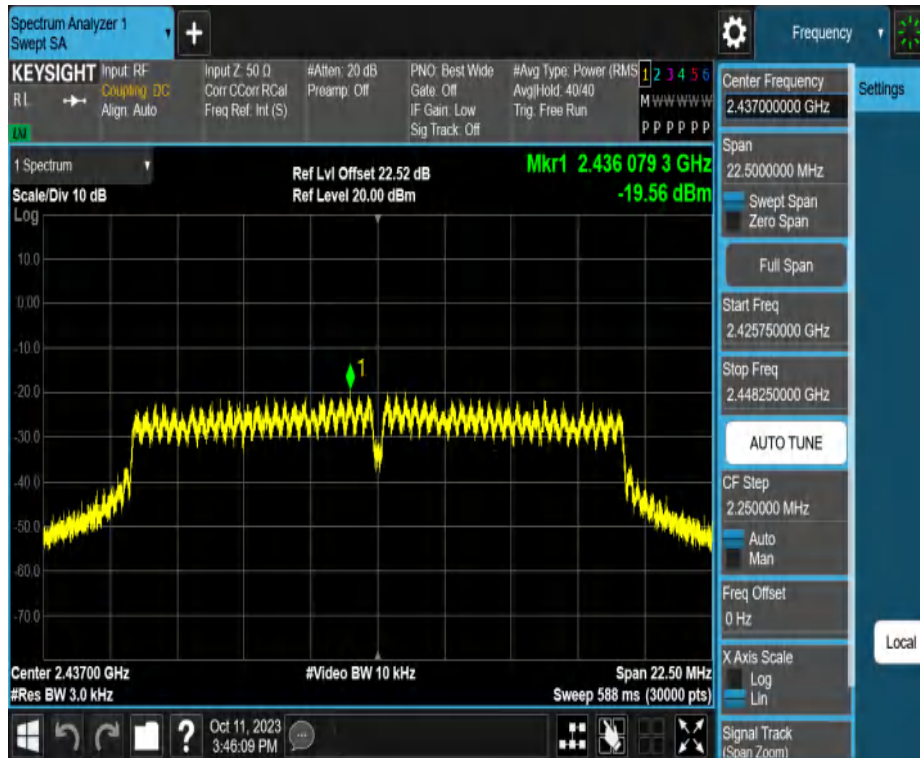
11G-CDD_Ant2_2437
