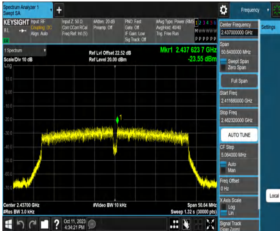
11N40MIMO_Ant2_2437
