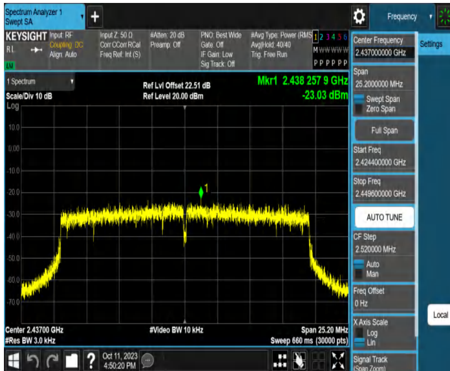
11AX20MIMO_Ant2_2437
