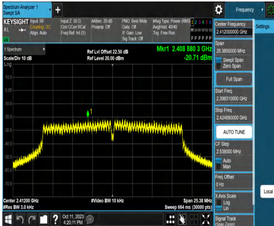
11N20MIMO_Ant2_2412
