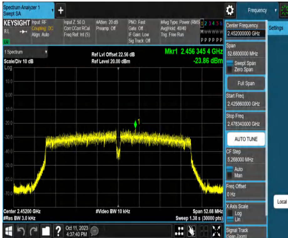
11N40MIMO_Ant2_2452
