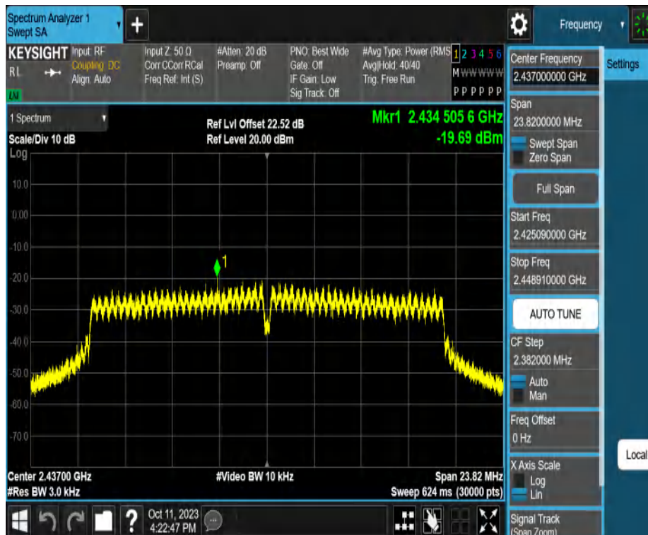
11N20MIMO_Ant2_2437
