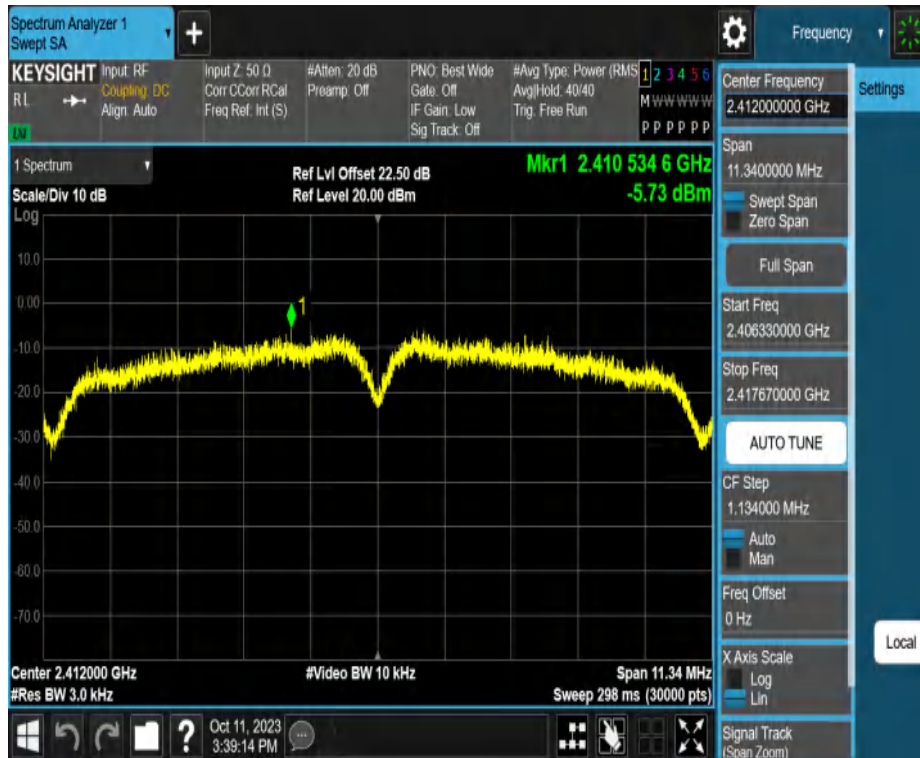
11B-CDD_Ant2_2412
