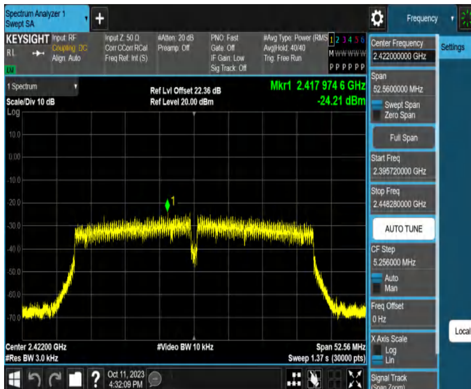
11N40MIMO_Ant2_2422
