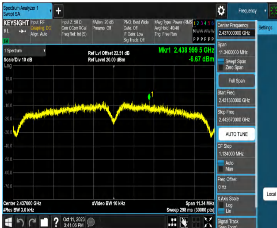
11B-CDD_Ant2_2437
