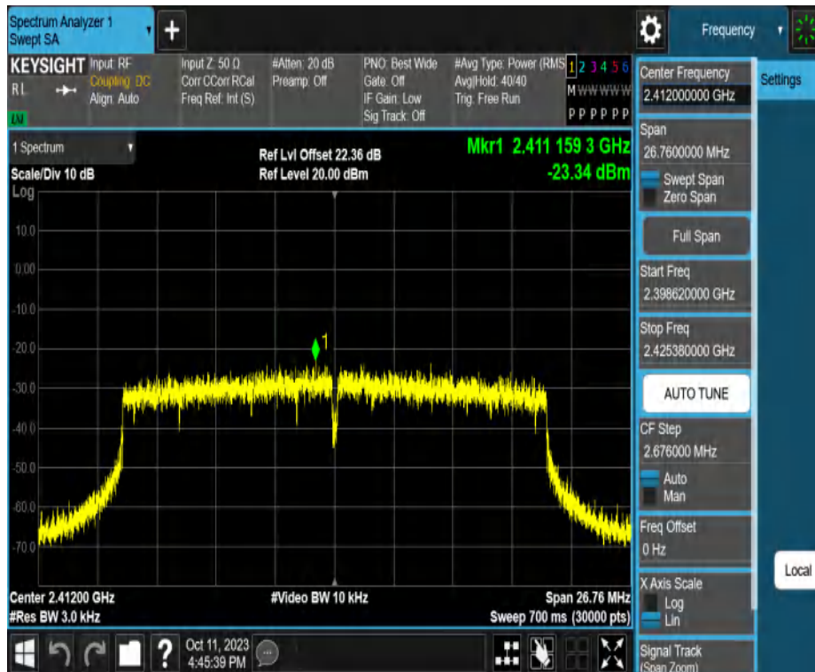
11AX20MIMO_Ant2_2412
