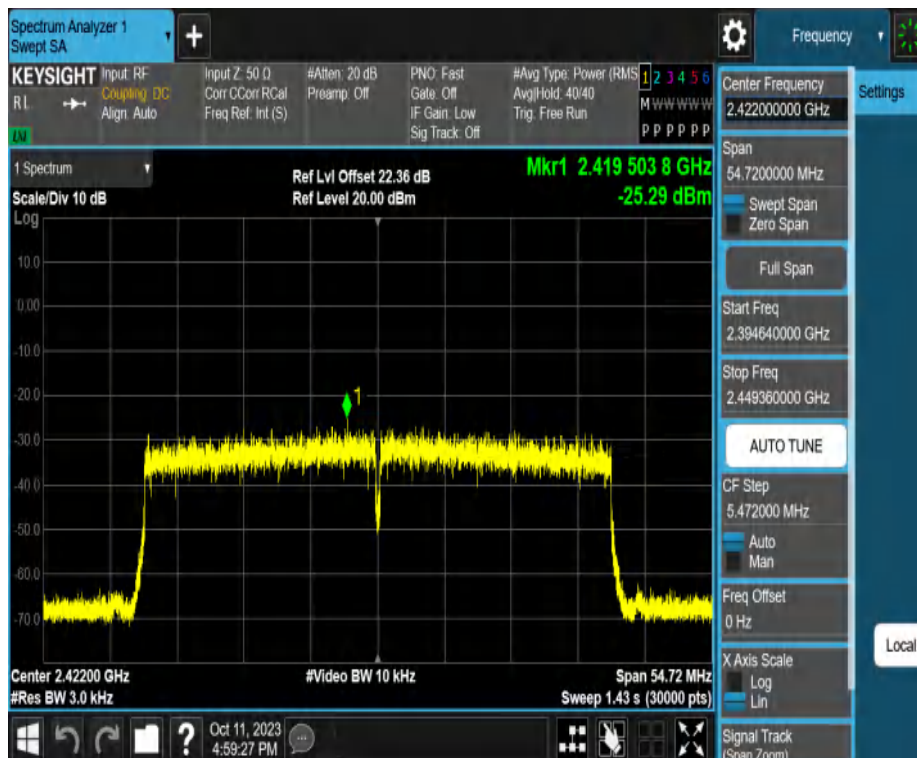
11AX40MIMO_Ant2_2422
