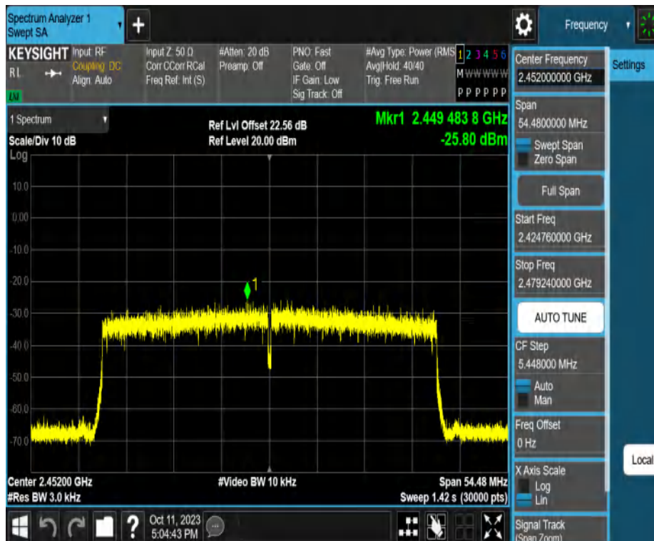
11AX40MIMO_Ant2_2452
