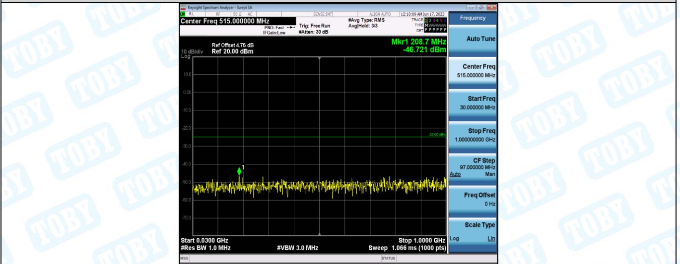
Band41-5MHz-QPSK-40215-1RB#0-Range1:30~1000MHz
