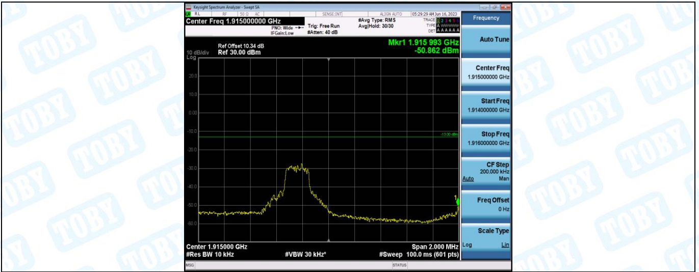
Band25-3MHz-QPSK-26675-1RB#14
