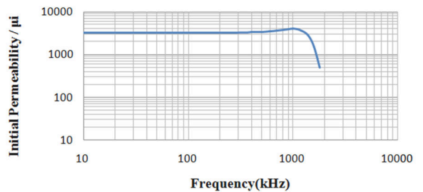
\mu_i -f
