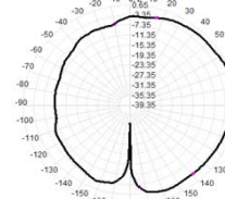
2480.0MHz Total(E2-YZ), Max: -0.14dB
