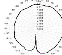
2500.0MHz Total(E2-YZ), Max: -1.00dB
