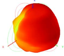
2500.0MHz H+V, ER: 40.6%
