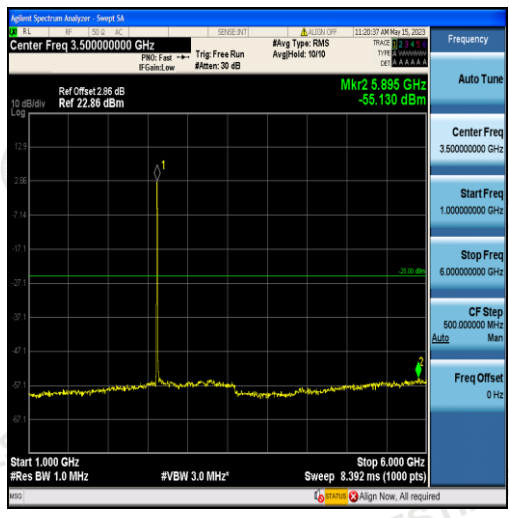
Band38-5MHz-QPSK-38225-25RB#0-Range2:1000~6000MHz
