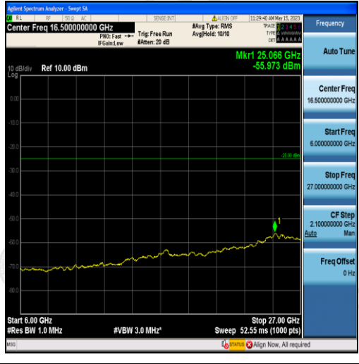
Band38-10MHz-QPSK-38000-50RB#0-Range3:6000~27000MHz
