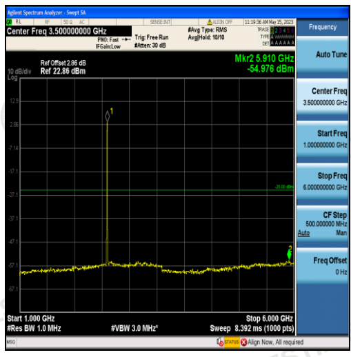
Band38-5MHz-QPSK-38000-25RB#0-Range2:1000~6000MHz
