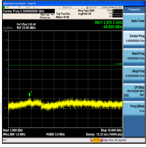
Band5-10MHz-QPSK-20525-50RB#0-Range2:1000~10000MHz
