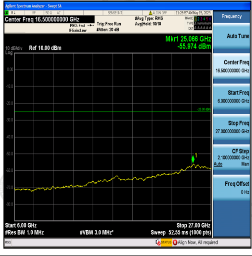
Band38-10MHz-QPSK-37800-50RB#0-Range3:6000~27000MHz
