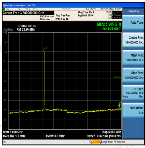
Band38-10MHz-QPSK-38000-50RB#0-Range2:1000~6000MHz
