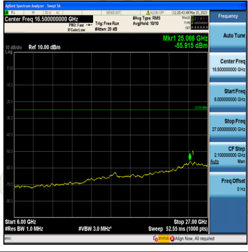
Band38-5MHz-QPSK-38225-25RB#0-Range3:6000~27000MHz
