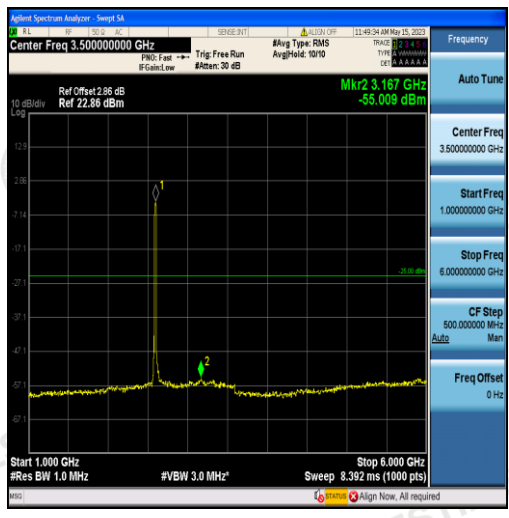
Band38-20MHz-QPSK-38000-100RB#0-Range2:1000~6000MHz
