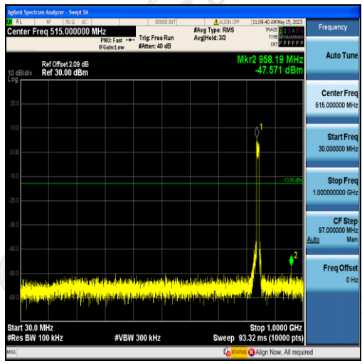
Band5-10MHz-QPSK-20600-50RB#0-Range1:30~1000MHz
