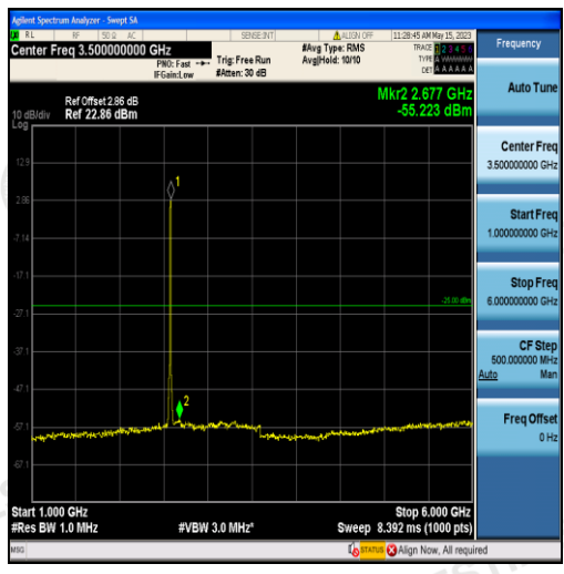
Band38-10MHz-QPSK-37800-50RB#0-Range2:1000~6000MHz
