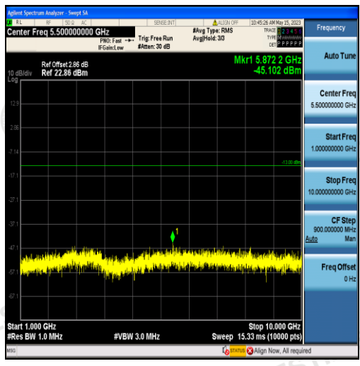
Band5-3MHz-QPSK-20415-15RB#0-Range2:1000~10000MHz
