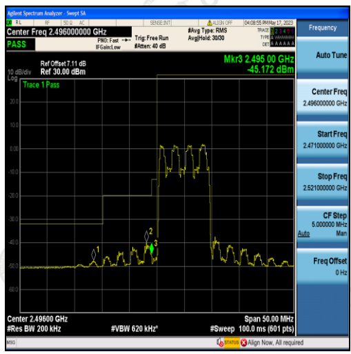
Band41-10MHz-QPSK-39700-50RB#0
