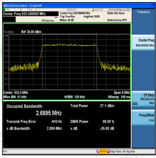
Band5-3MHz-QPSK-20415-15RB#0-2.6895
