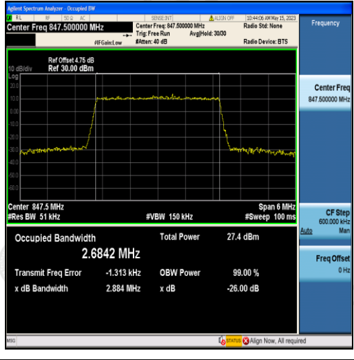
Band5-3MHz-QPSK-20635-15RB#0-2.6842
