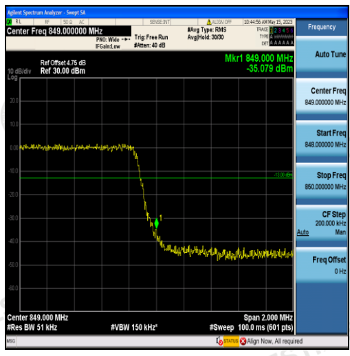
Band5-3MHz-QPSK-20635-15RB#0
