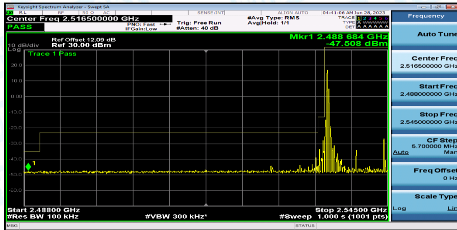
Band41_Band41_10MHz_QPSK_40090_1RB#0
