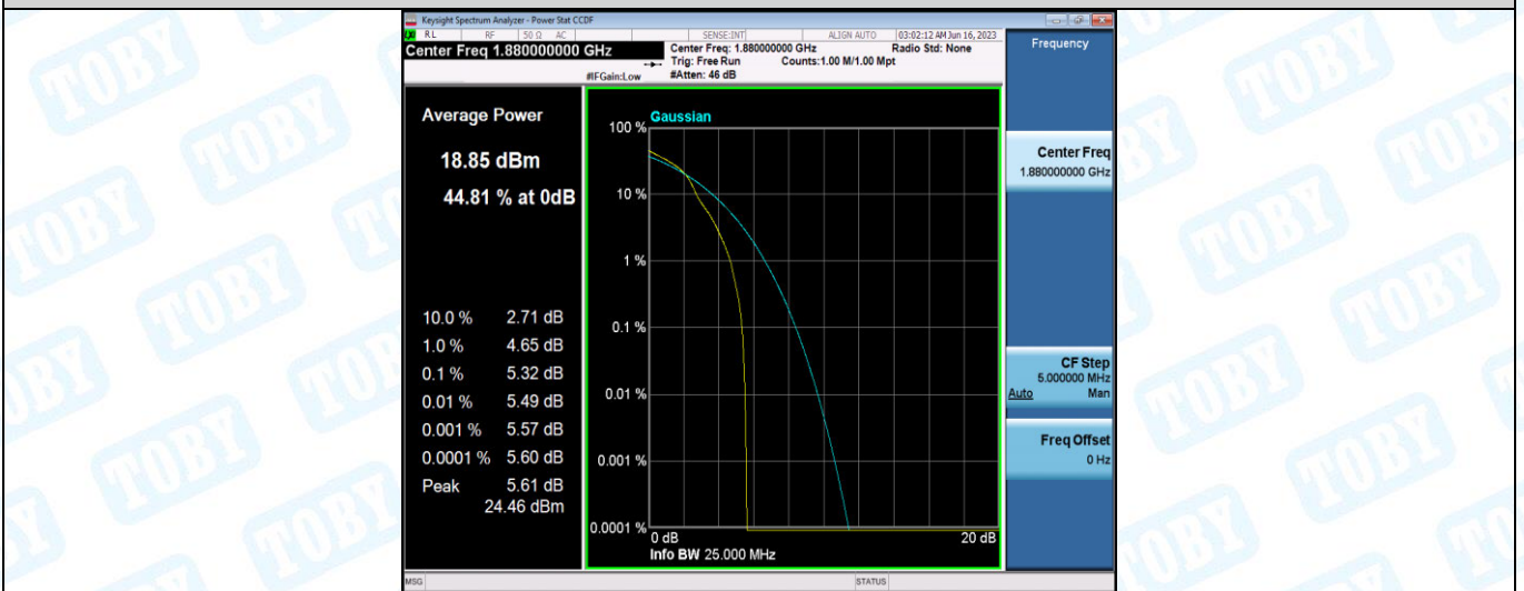
Band2-20MHz-16QAM-18900-27RB#0
