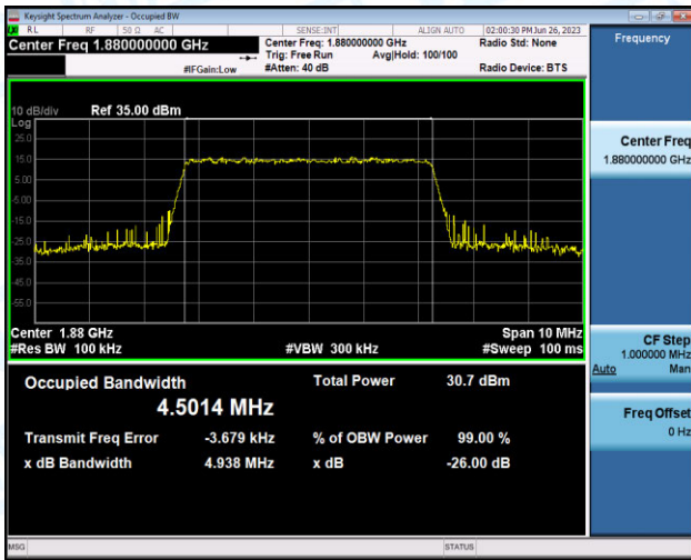
Band2-5MHz-QPSK-18800-25RB#0-PASS
