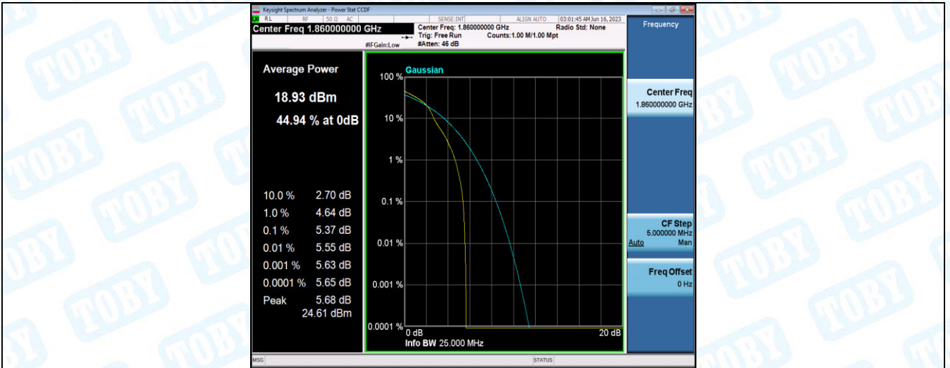
Band2-20MHz-16QAM-18700-27RB#0
