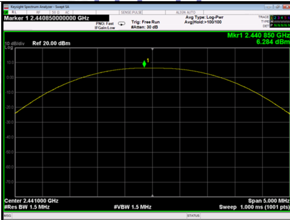
GFSK DH5 MCH 2441MHz Ant1 NTN
