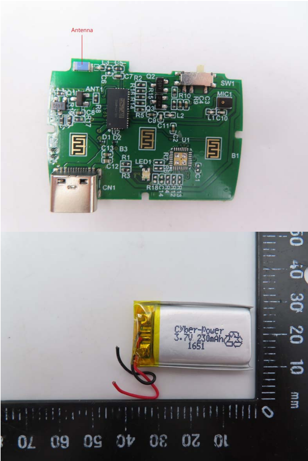
Antenna
