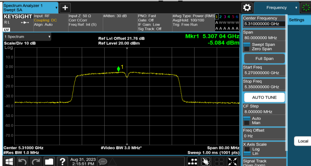
11N40MIMO Ant2 5310
