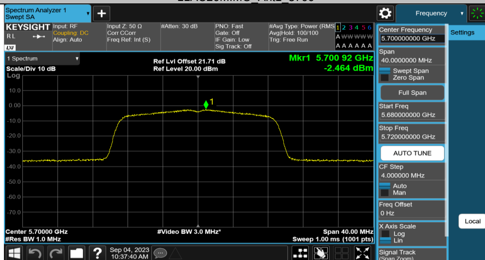
11AC20MIMO_Ant2_5700
