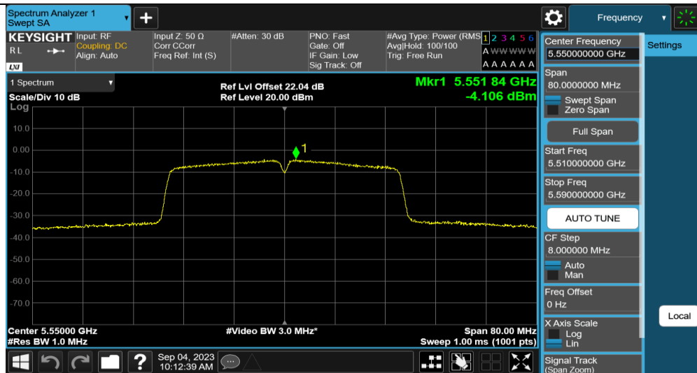
11N40MIMO Ant2 5550
