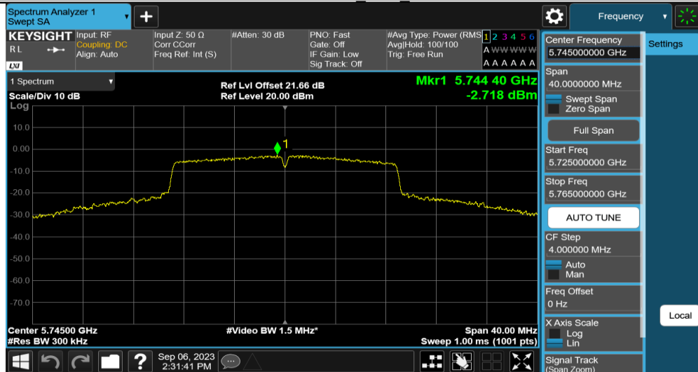
11N20MIMO Ant2 5745
