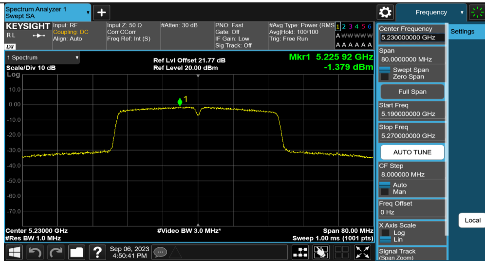
11N40MIMO Ant2 5230
