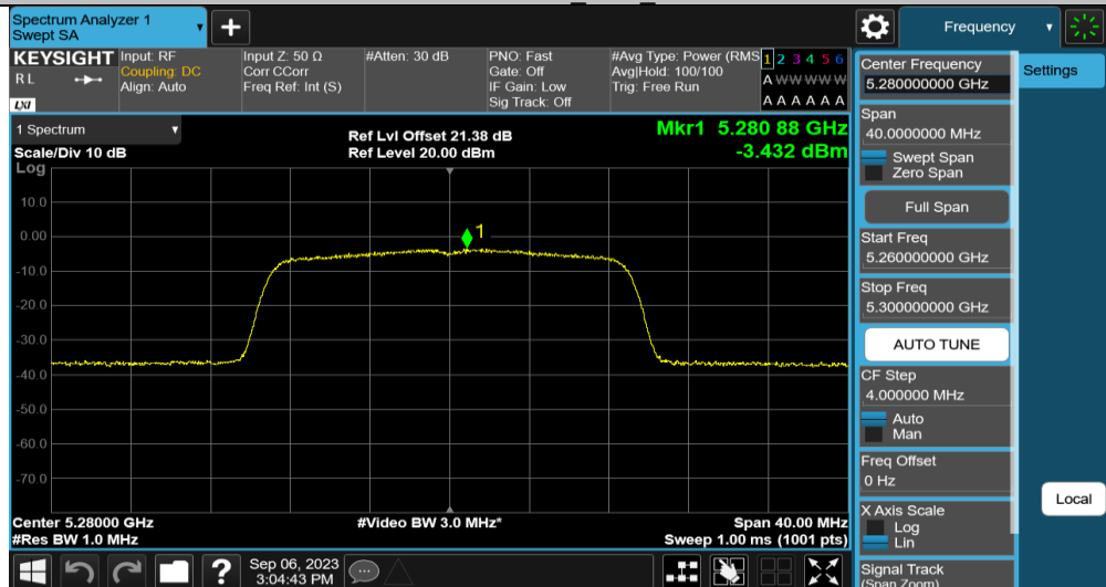
11AC20MIMO_Ant2_5280
