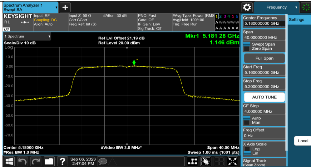
11AC20MIMO_Ant2_5180
