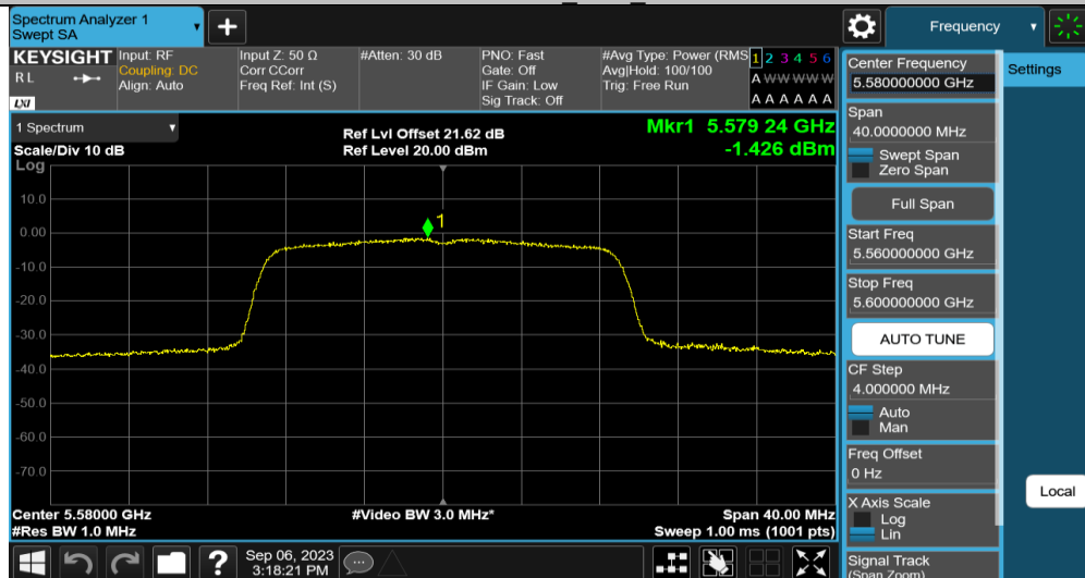
11AC20MIMO_Ant2_5580
