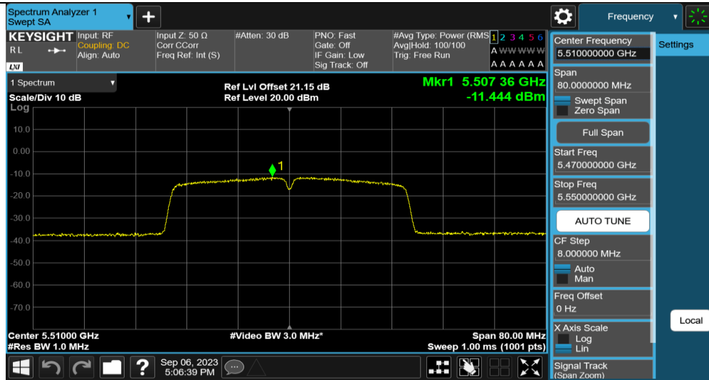
11N40MIMO Ant2 5510
