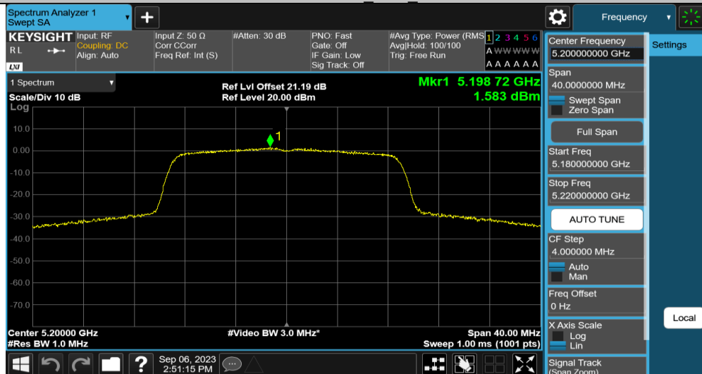
11AC20MIMO_Ant2_5200
