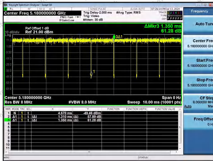
NTVN-11AC20SISO-Ant1-5180
