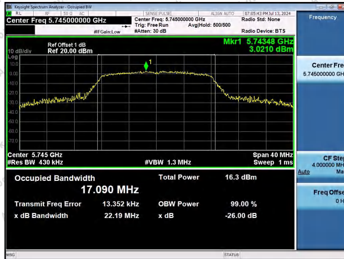
11A-Ant1-5745
