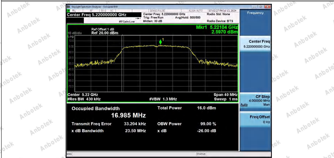
11A-Ant1-5220
