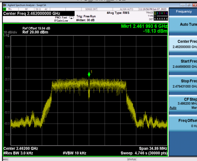
11G_Ant1_2462
