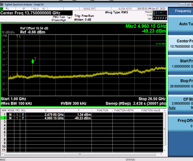
BLE_1M_Ant1_2480_1000~26500
