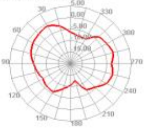
5849.994MHz E1
