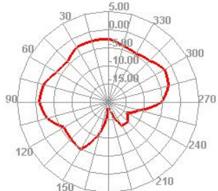
5849.994MHz E2
