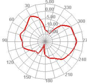
5421.426MHz E1
