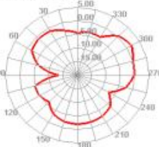
5528.568MHz H
