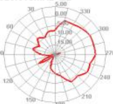
5528.568MHz E2
