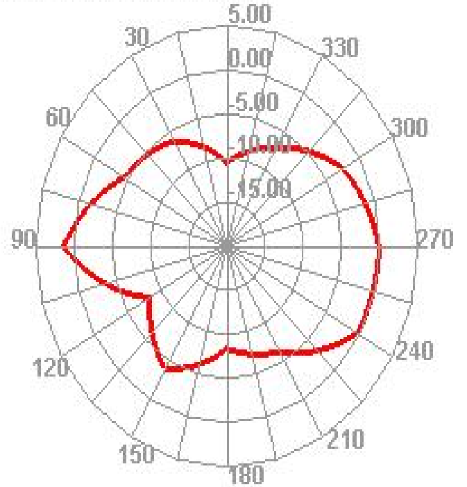
2400.000MHz H
