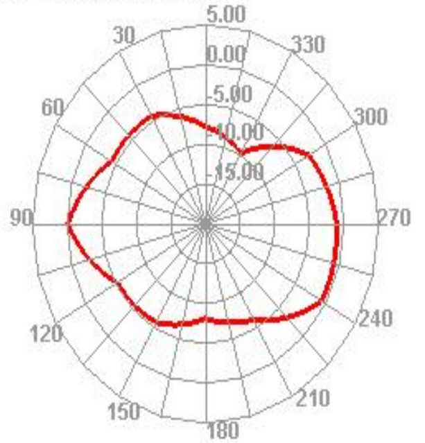
2500.000MHz H
