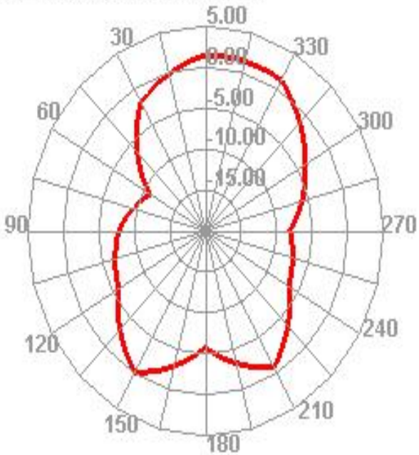
2500.000MHz E1
