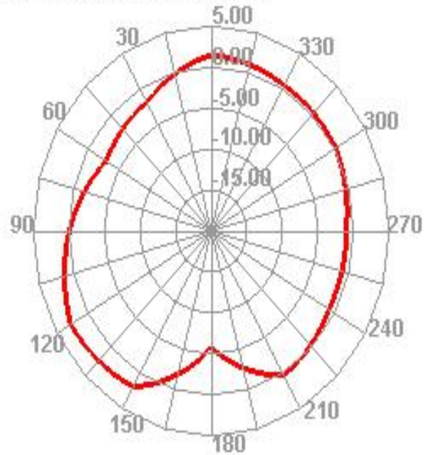
2500.000MHz E2
