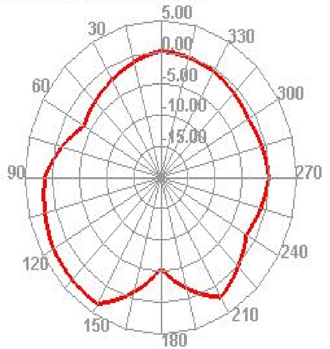
2400.000MHz E2
