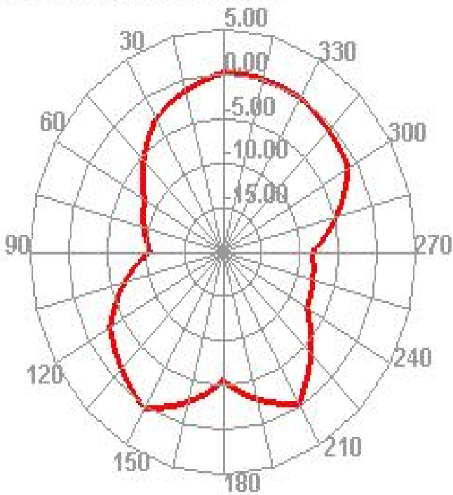
2400.000MHz E1
