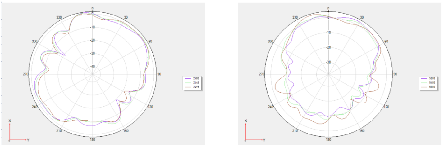
Theta 90 2D图
