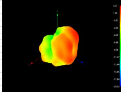
5500MHz
