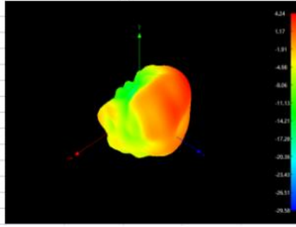
5000MHz
