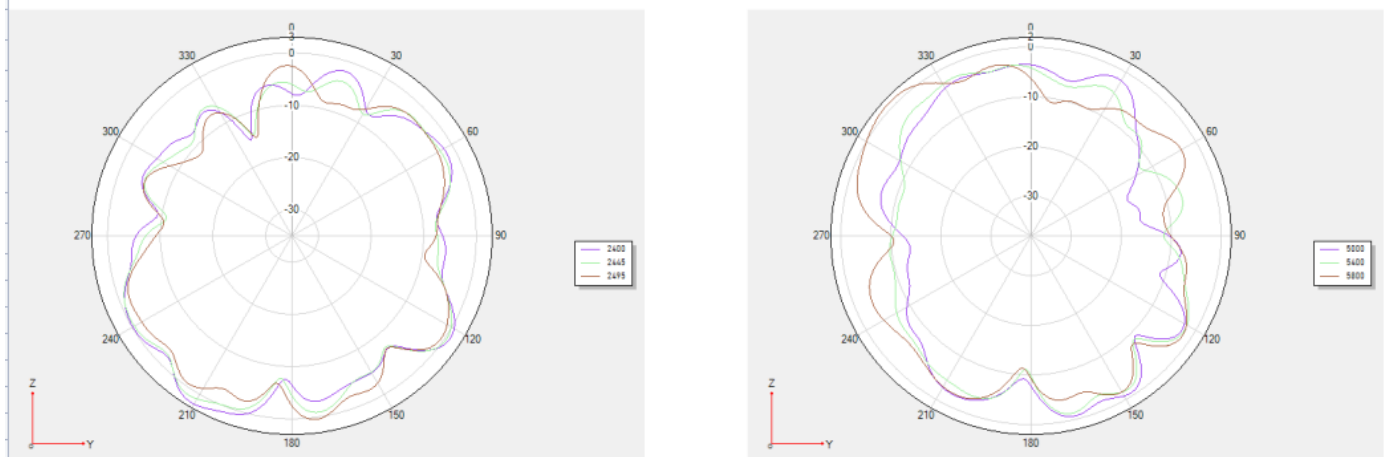
Phi 90 2D图
