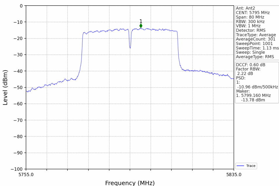
802.11n(HT40)_HCH_5795MHz_Ant2_NTNV
