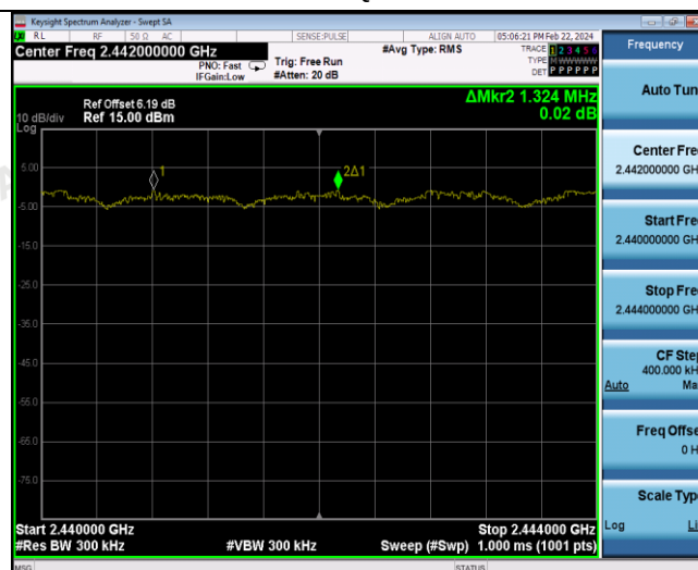
8DPSK
